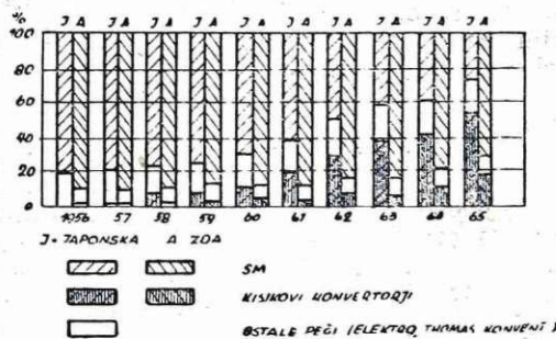
Letna proizvodnja surovega jekla v različnih proizvodnih agregatih na Japonskem in v ZDA
