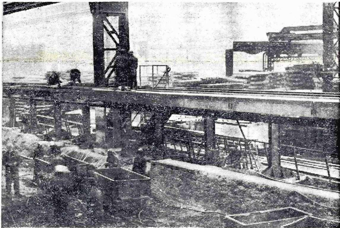
V livni jami martinarne nadaljujejo z gradnjo podesta
