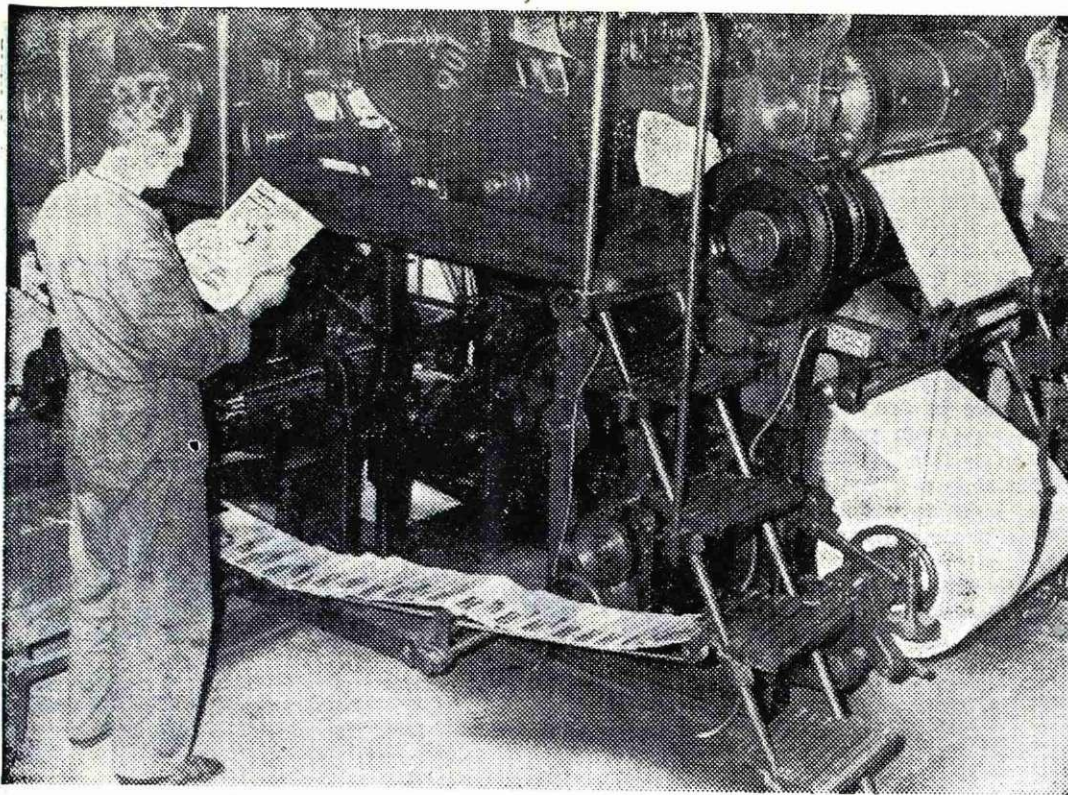
Rotacijski stroj. Strojnik si ogleduje prve izvode. Morda bo treba še kaj popraviti
