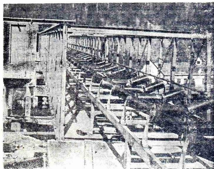
Železno ogrodje je nameščeno, manjka le še transportni trak
