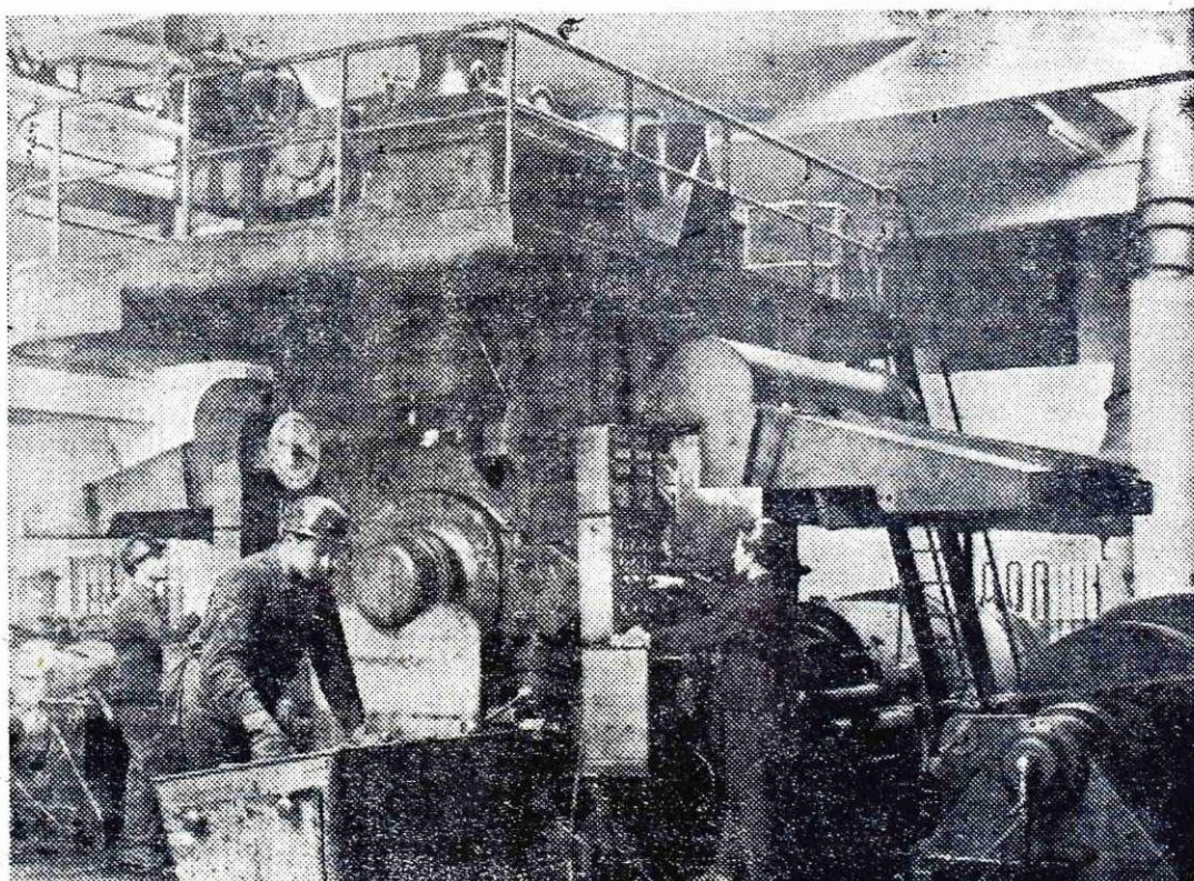
Valjčno ogrodje Siemag v hladni valjarni
