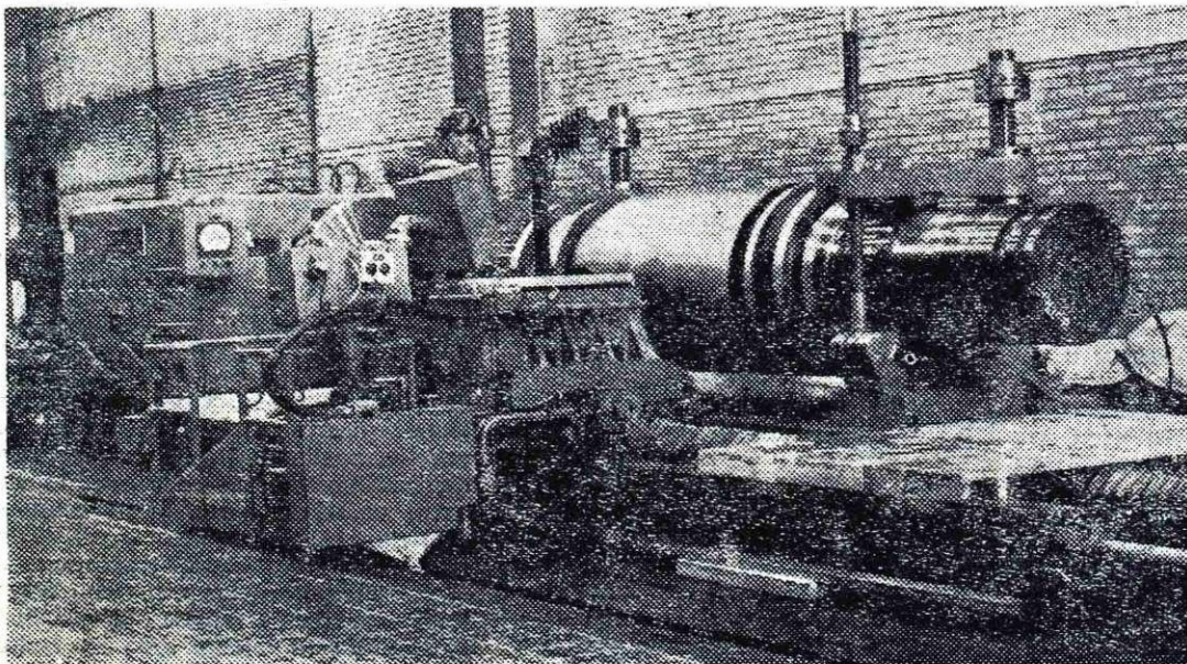
Stružnica Blaw-Knox Medart, za struženje valjev za bluming
