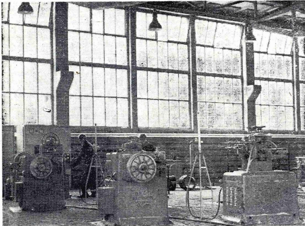
Nova patentirnica naglo spreminja podobo. Nameščeni so že številni stroji. Na zgornji sliki so že nameščeni angleški žičarski stroji firme DECO, spodaj pa navijalna vretena patentirne proge
