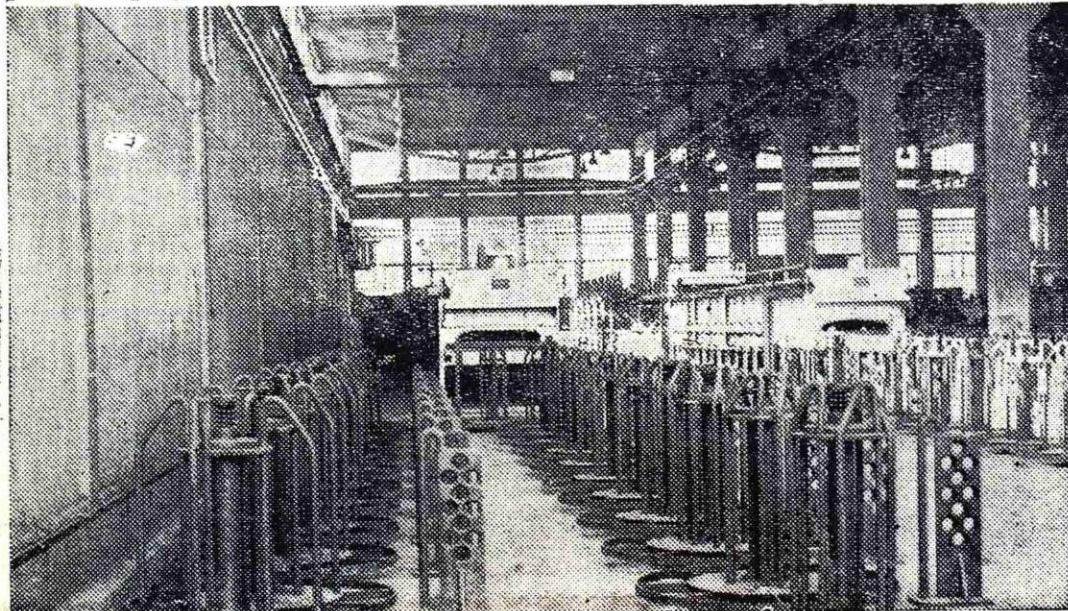
Nova patentirnica naglo spreminja podobo. Nameščeni so že številni stroji. Na zgornji sliki so že nameščeni angleški žičarski stroji firme DECO, spodaj pa navijalna vretena patentirne proge
