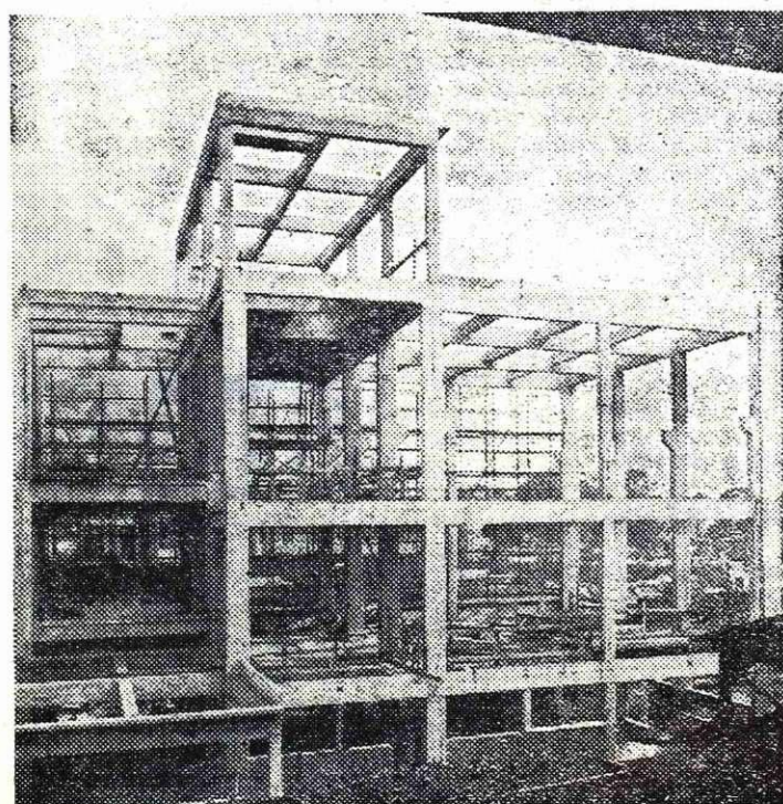
Betonski skelet drobilnice I.
