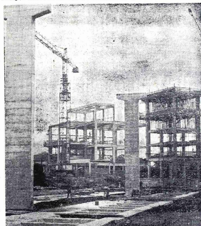
Pod temi stebri bo tekel transportni trak za koks
