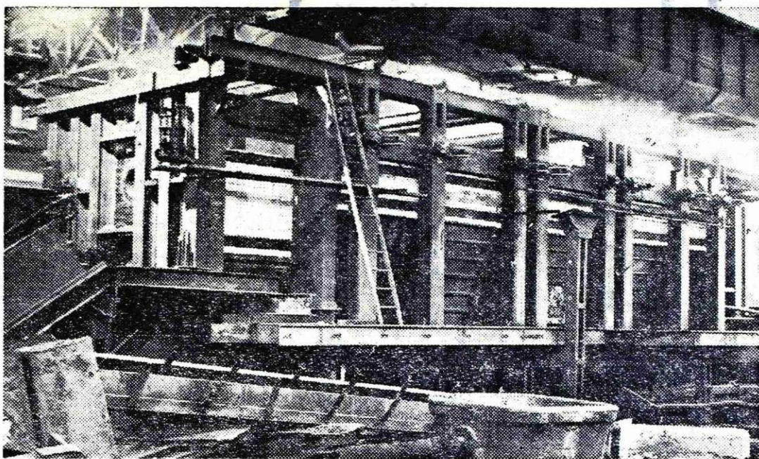
Sedma SM peč, ali peč V, med remontom
