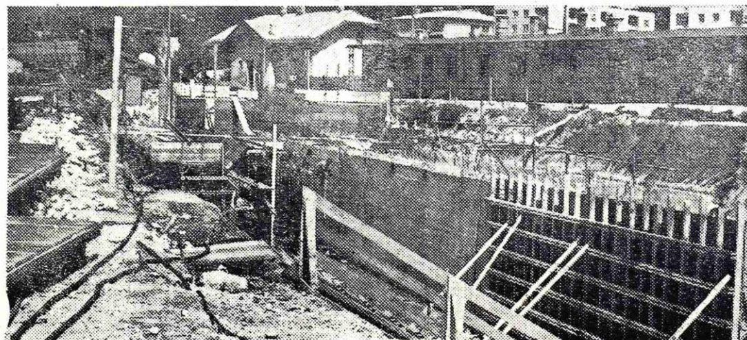
Betoniranje 100-metrskega rova v novem skladišču koksa
