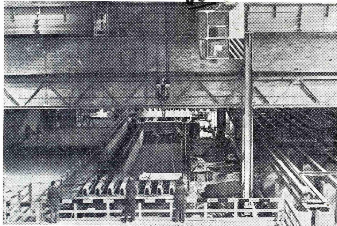
Zerjav bo prenesel iz 8-tonski bram valjane slabe v skladišče odkoder jih bodo s kamionom prepeljali v valjarno 2400
