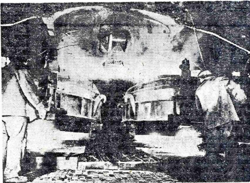
Naprava za kontinuirano vlivanje v Donecku ima zmogljivost 550.000 ton jekla letno. Slaba stran tega načina vlivanja jekla je v tem, da danes odlivajo po tem postopku lahko le okoli 30 vrst kvalitetnega jekla, ki vsebuje od 0,1 do 0,3 % ogljika.
