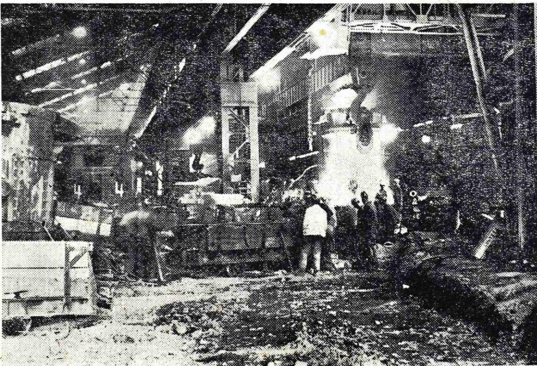
V livni jami martinarne so začeli postavljati normalni tir, da bi lahko prešli na vlivanje jeklenih blokov na vozovih
