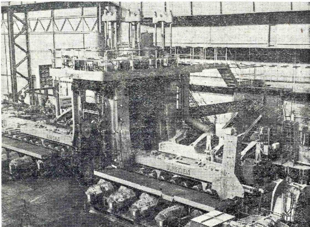
Vročo bramo bodo kmalu stisnili vrteči se valji
