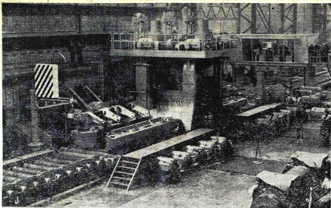
Valji novega bluminga so stisnili žareč jeklen blok — bramo
