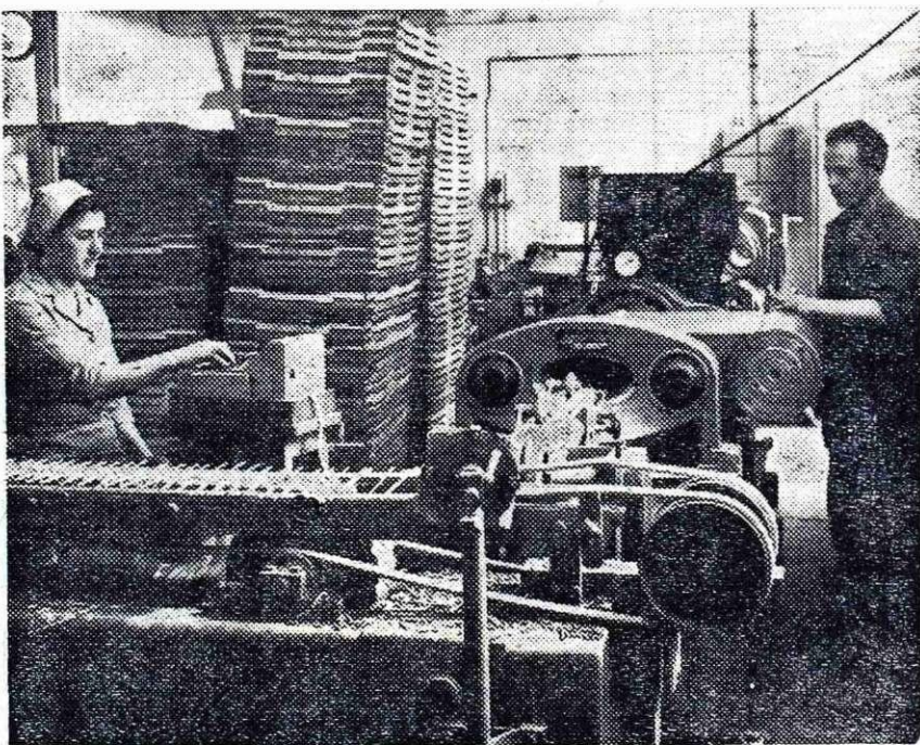
V naši železarni izdelujemo tako imenovane gole in oplasčene elektrode. Na sliki je stiskalnica, kjer nanesejo na golo elektrodo posebno maso ali »plaseč«.
