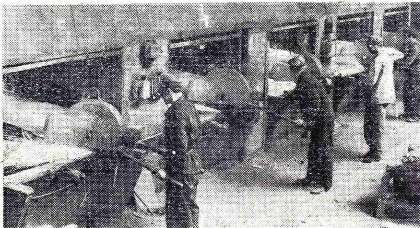
Čiščenje površine gredic (valjarniškega izdelka kvadratne oblike) z brušenjem
