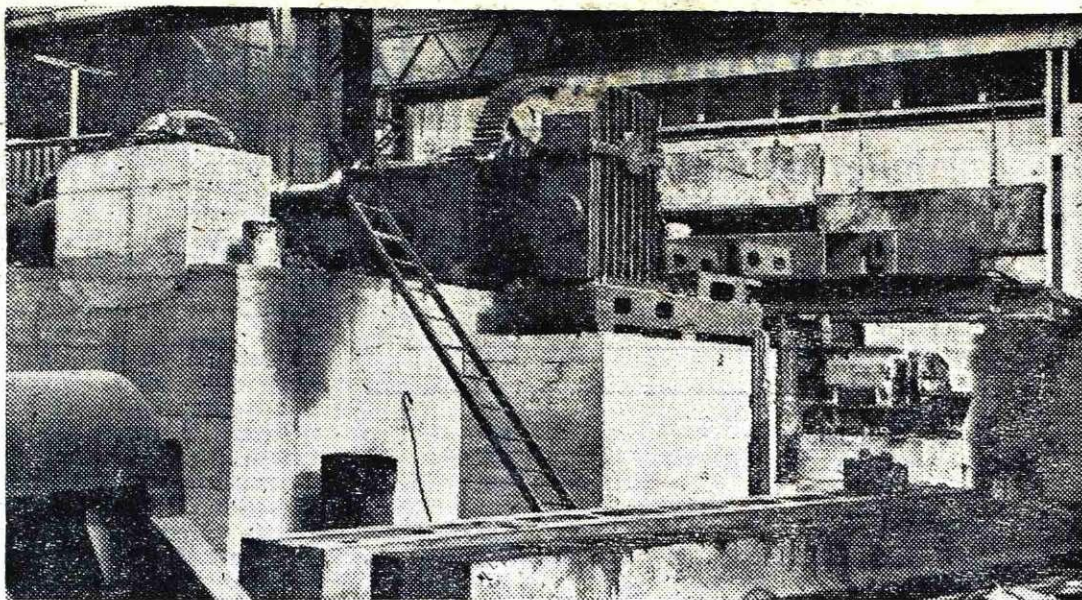
Del potisne peči v novi valjarni Bela
