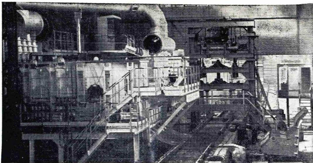
Potisna peč v novi valjarni Bela
