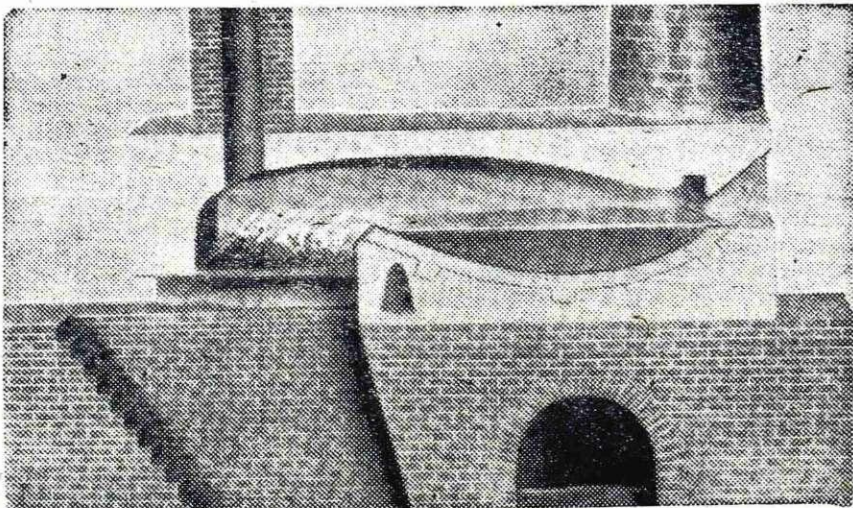
Prerez skozi pudlovko
