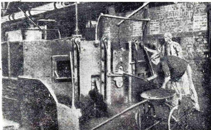
Pudlovka, kurili so jo s premogom, okoli 1. 1860
