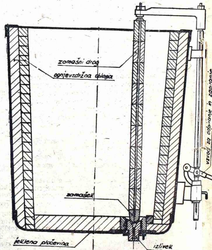
Prerez skozi ponovco za vlivanje surovega jekla
