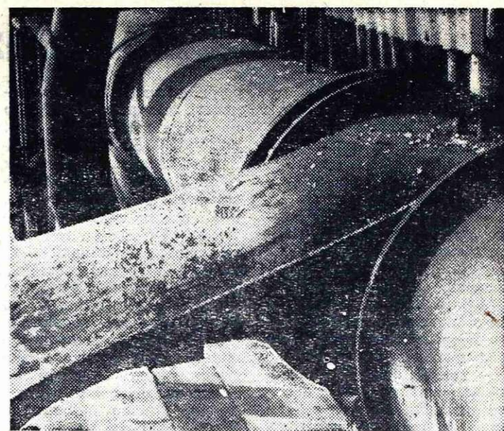
Del raztrgane cevi za zrak pri plinskih generatorjih
