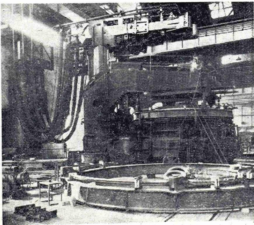
Obločna električna peč ASEA v naši železarni
