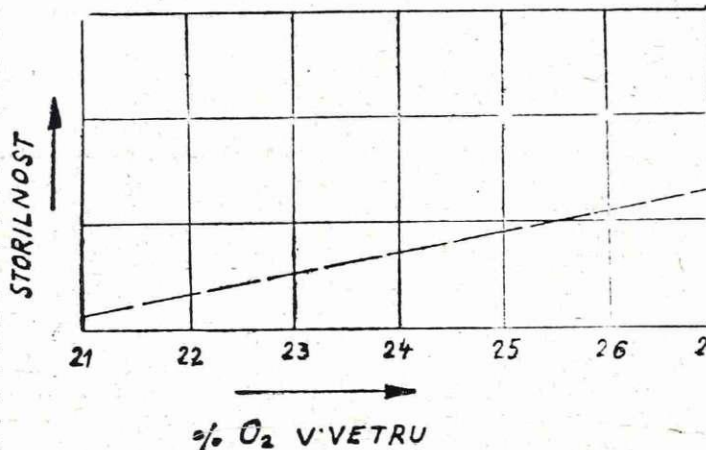
Povečanje storilnosti z dodajanjem kisika zraku
