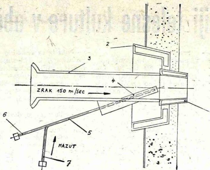
Pihalica za dodajanje mazuta v plavž
