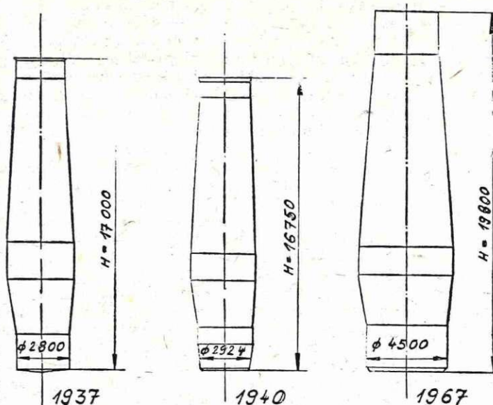
Skica sedanjih in bodočega plavža
