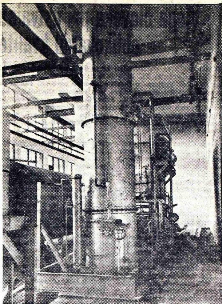
Generator za proizvodnjo zaščitnega plina (Novi jeklovlek)
