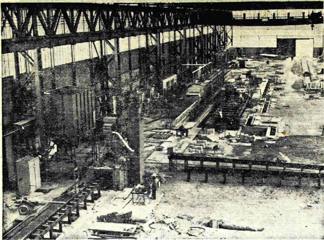
Pogled na novi jeklovlek z žerjava. V teku so priprave za prvo vrtenje na posameznih napravah.
