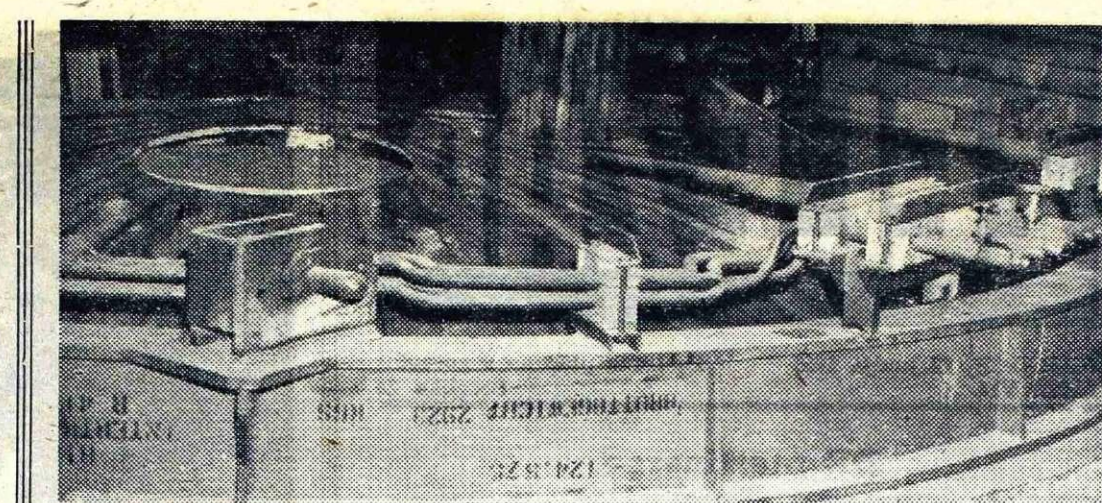
Obok za novo ASEA električno peč, ki se je zelo dobro obnesel
