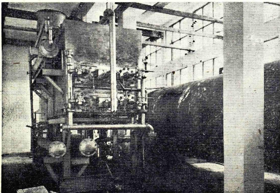
Generator za proizvodnjo zaščitnega Rx plina
