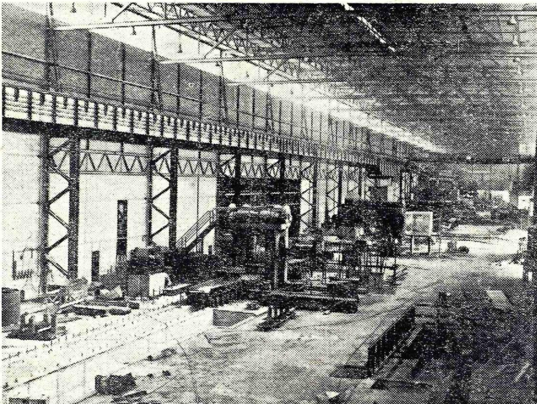
Pogled na bluming in steckel valjarno. Dela bi lahko hitreje napredovala, če bi dobavitelji domače opreme izpolnili pogodbene obveznosti.
