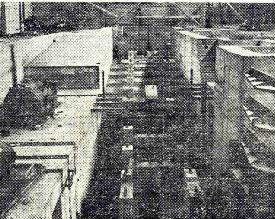
Pogled na bluming in steckel valjarno. Dela bi lahko hitreje napredovala, če bi dobavitelji domače opreme izpolnili pogodbene obveznosti.
