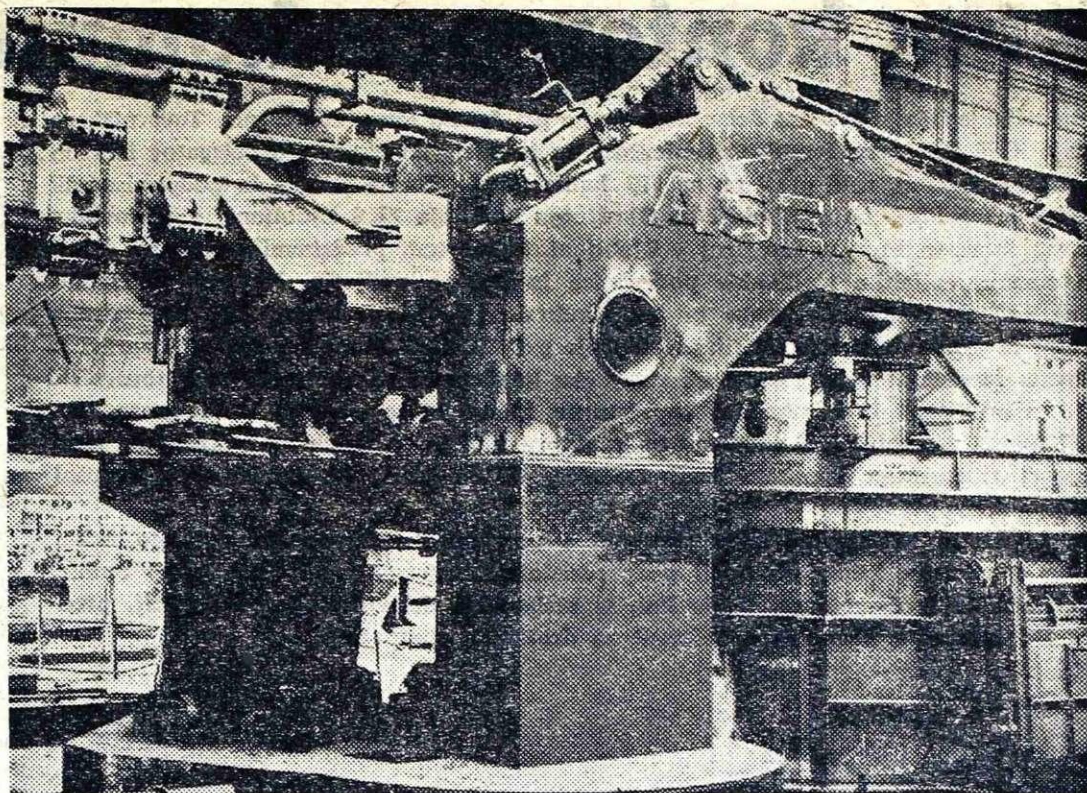
Nova 60-tonska ASEA električna peč bo kmalu nared za obratovanje
