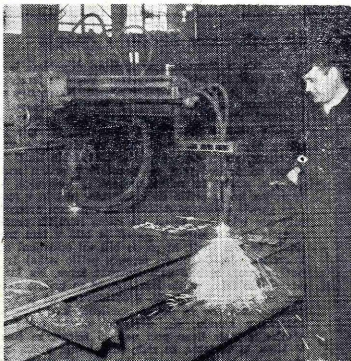
Za 80 % se je povečala storilnost sektorja v adjustaži valjarne 2400, ko so Jože Volman, Anton Dežman in Janez Štagar izdelali in namestili še drugi gorilec
