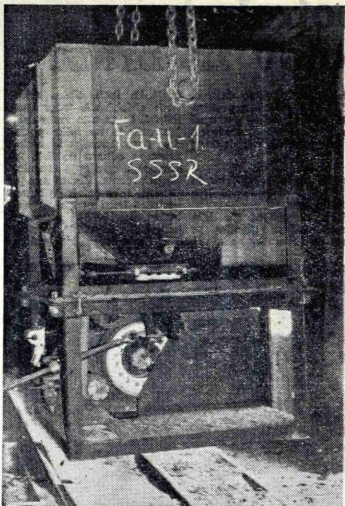
Stroj za zametavanje SM peči s sintermagnezitom
