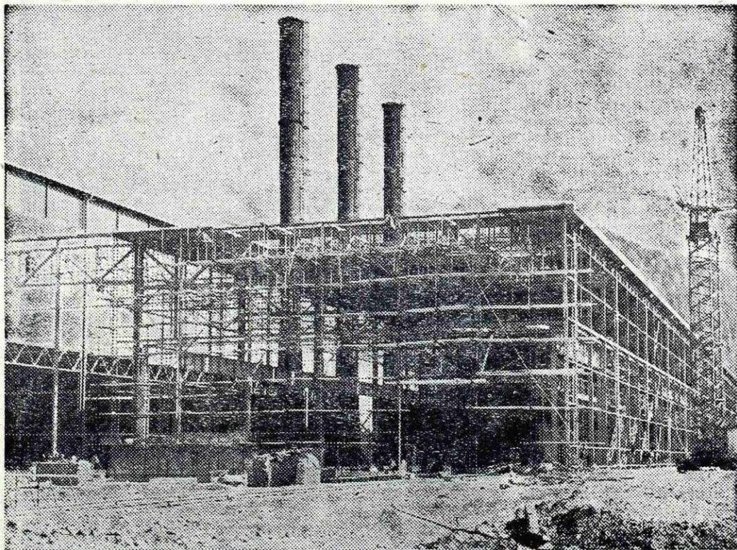
Med gradnjo hale za težko progo na Belškem polju
