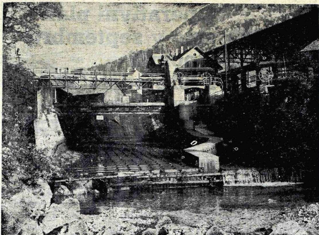
Naprave na jazu bo treba dopolniti s čistilnimi napravami. Reportažo o delovni enoti plinske in vodne energije berite na srednji strand
