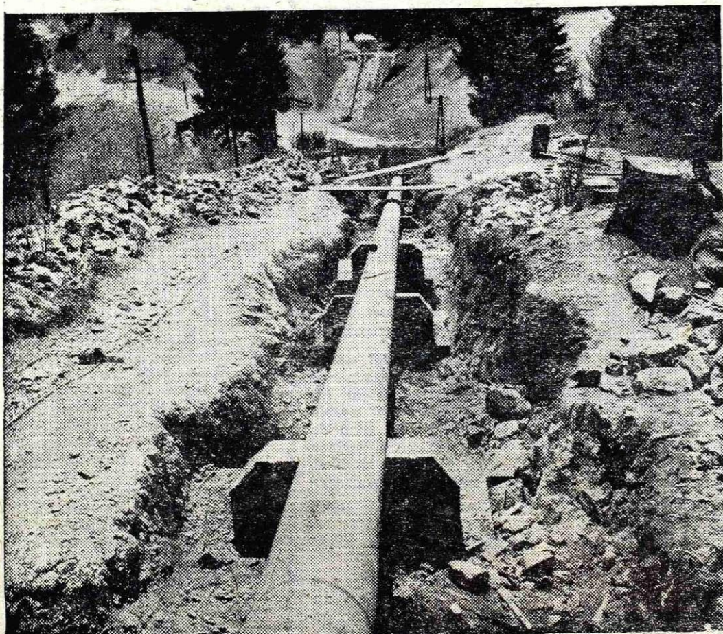
Visokotlačni cevovod, ki je speljan iz Javorniškega rovta je star preko 60 let, zato so ga morali obnoviti
