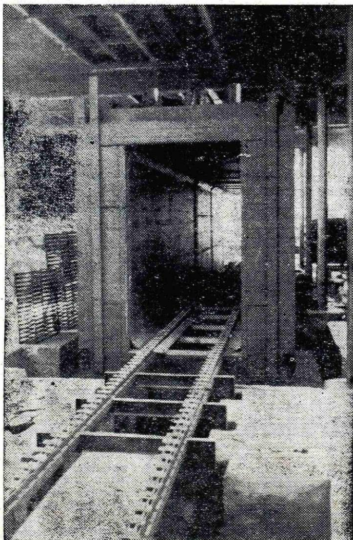
V elektrodnem oddelku so začeli z montažo nove sušilne peči. Konstrukcijo te peči so pred kratkim pripeljali iz Italije
