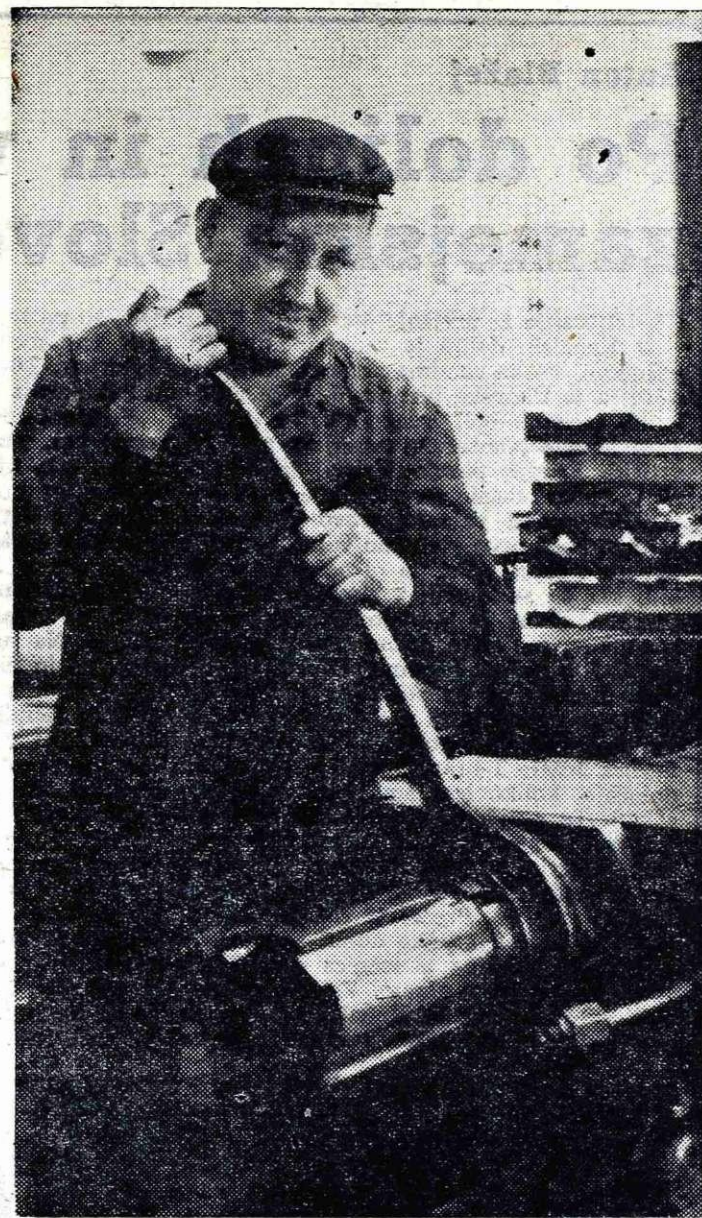
Anton Arh, ključavničar v hladni valjarni-žičarni, je izdelal posebno stojalo, ki omogoča kar najbolj natančno montažo para delovnih valjev.
