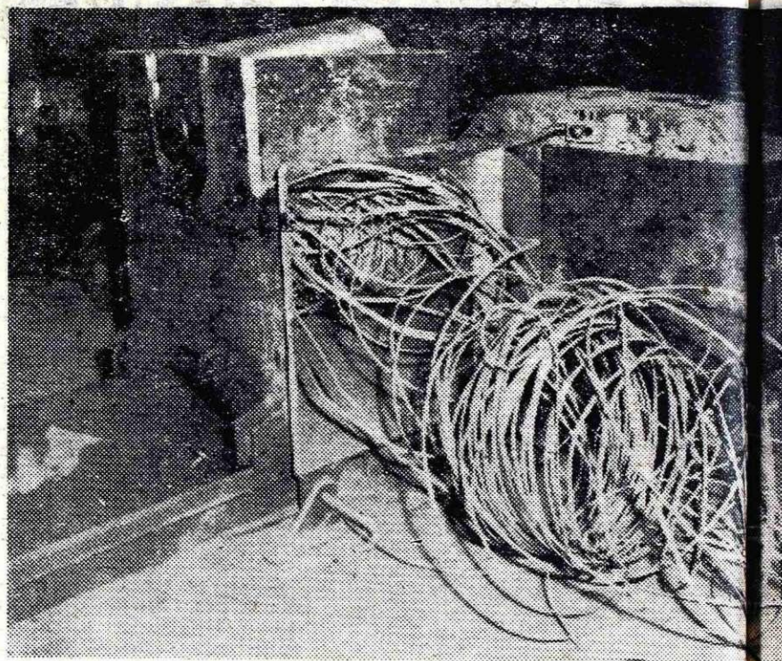
Nov stroj za navijanje rene v žični valjarni. Po vzorcu iz Železarne Zaso inž. Sekne, obratovodja Grošelj in tehniki Zupan, Kovač in Zorko.
