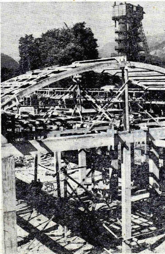
Na desnem bregu Save, tik pred železniškim mostom pa bo nova kisikarna
