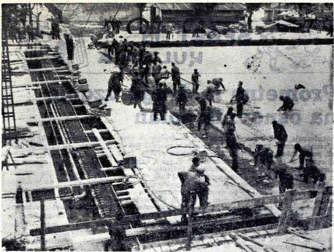
Betoniranje plošče iz prednapetega betona na drsalšču Podmežaklje je bilo zelo zahtevno. Delati so morali brez prekinitev.
