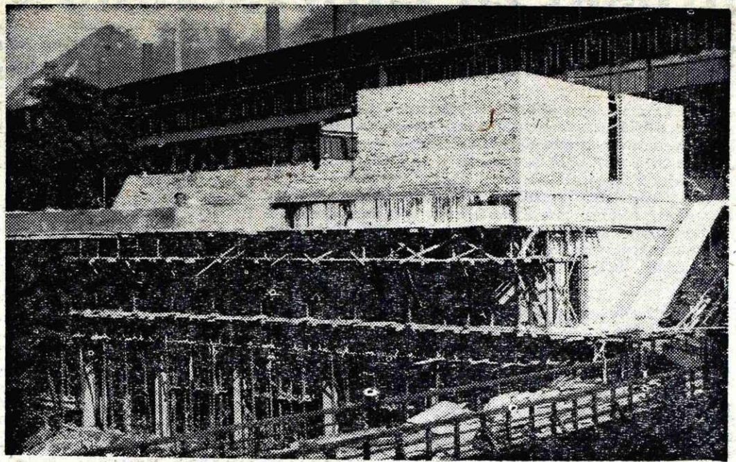
Na levem bregu Save, pod žično valjarno, gradimo novo RTP postajo
