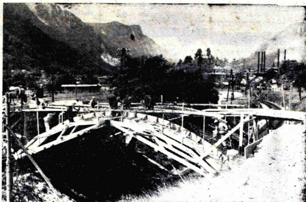
V torek so delavci gradbenega podjetja »Projekt« zabetonirali obok novega železniškega nadvoza pri osnovni šoli na Koroški Beli. Gradbena dela lepo napredujejo, zato lahko pričakujemo, da bo nadvoz zgrajen v predvidenem roku.
