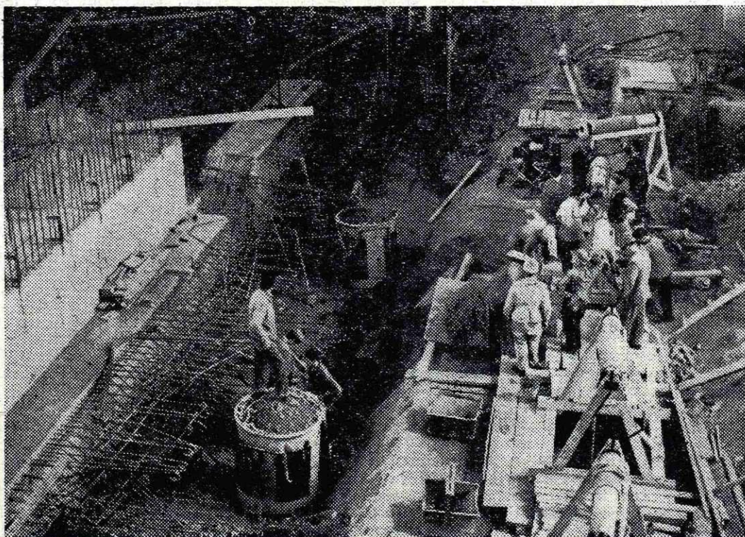
Gradbeni delavci v novih valjarnah na Belškem polju hitijo z deli, da bi čimveč zamenjali nadomestila
