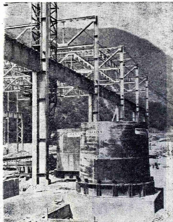
Na Belškem polju rastejo dimniki in se bo kmalu začelo kaditi
