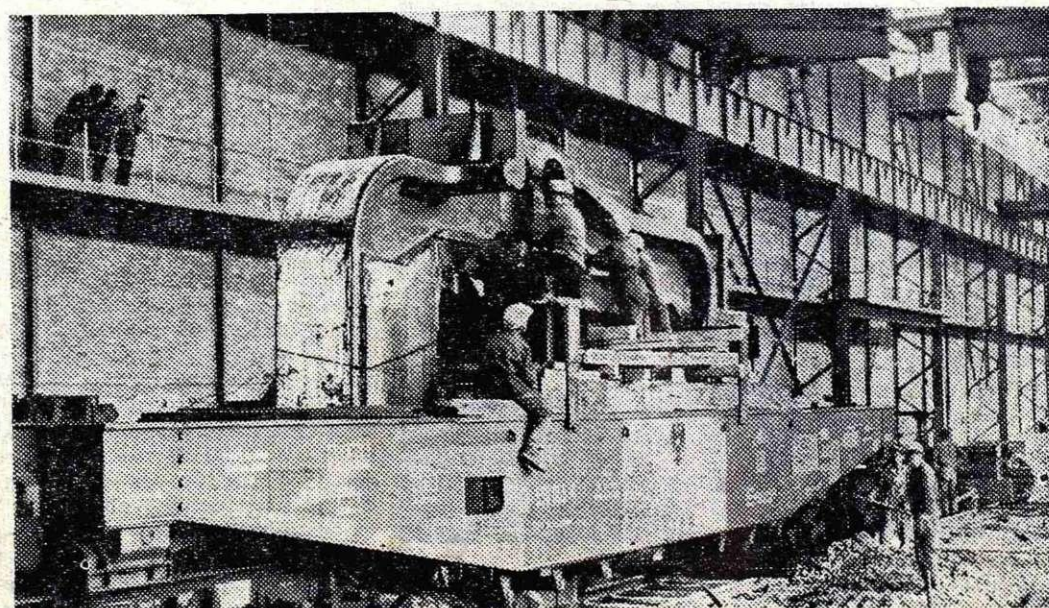
Blizu 120 ton tehta ta del stojala za novo bluming valjarno na Belškem polju, ki naj bi v letu 1965 že začela obratovati
