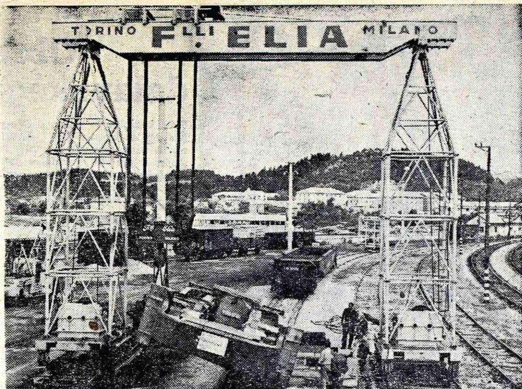
S posebnim dvigalom, ki so ga pripeljali iz Milana (Italija) so v Postojni pretovorili stojalo na železniški vagon
