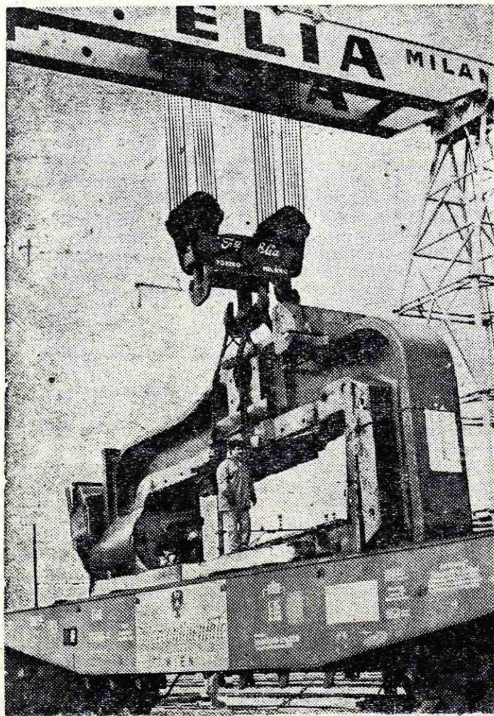
Zaradi neobičajne teže in velikosti je bil za transport stojala potreben poseben vagon
