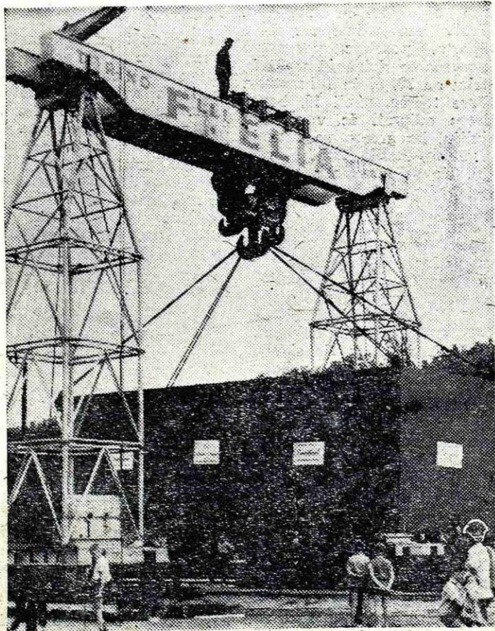
V Postojni so 49 ton težek del za kisikarno naložili na poposeben železniški vagon, s katerim ga bodo pripeljali na Jesenice
