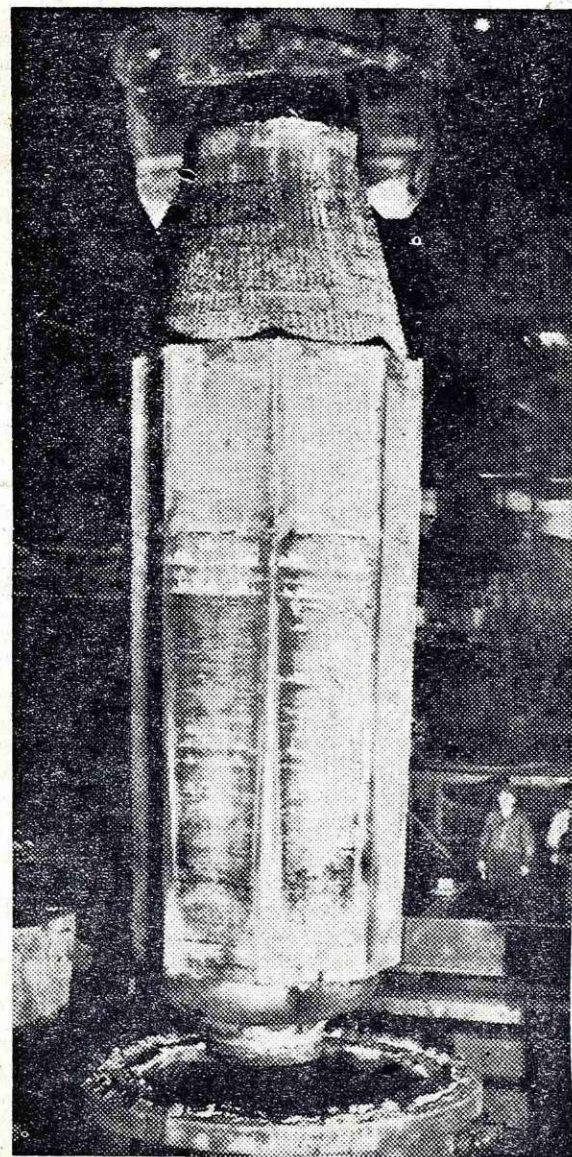
Velik 180-tonski ingot, kakršne odlivajo v třineški železarni
