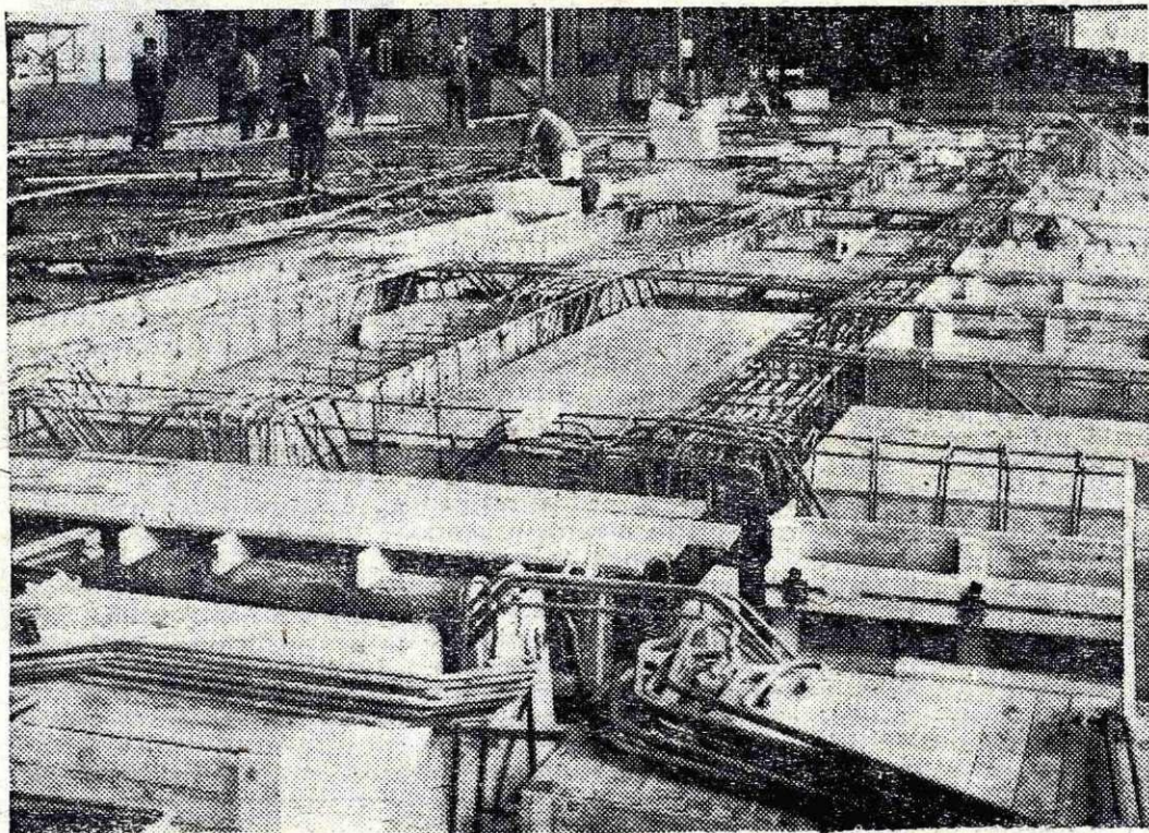
Gradnja temeljev za nove naprave
