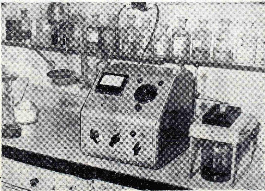
Prprava, ki jo v OTK uporablja za elektropolliranje metalo-grafskih vzorcev
