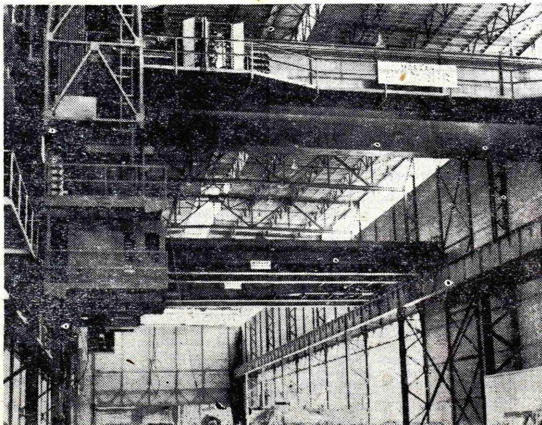
Montaža novega striper žerjava v valjarnah Bela na Belškem polju
