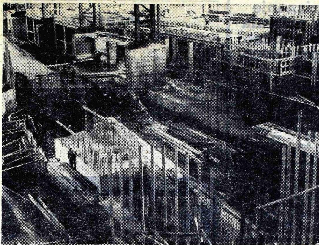
Z betoniranjem temeljev za strojne naprave na Belškem polju morajo zelo pohiteti, če hočejo, da bodo omogočili pravočasen začetek montaže strojev
