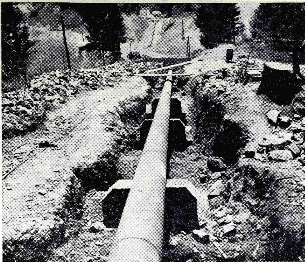
Visokotlačni cevovod, ki so ga položili v Javorniškem rovtu, je dolg 300 m.
