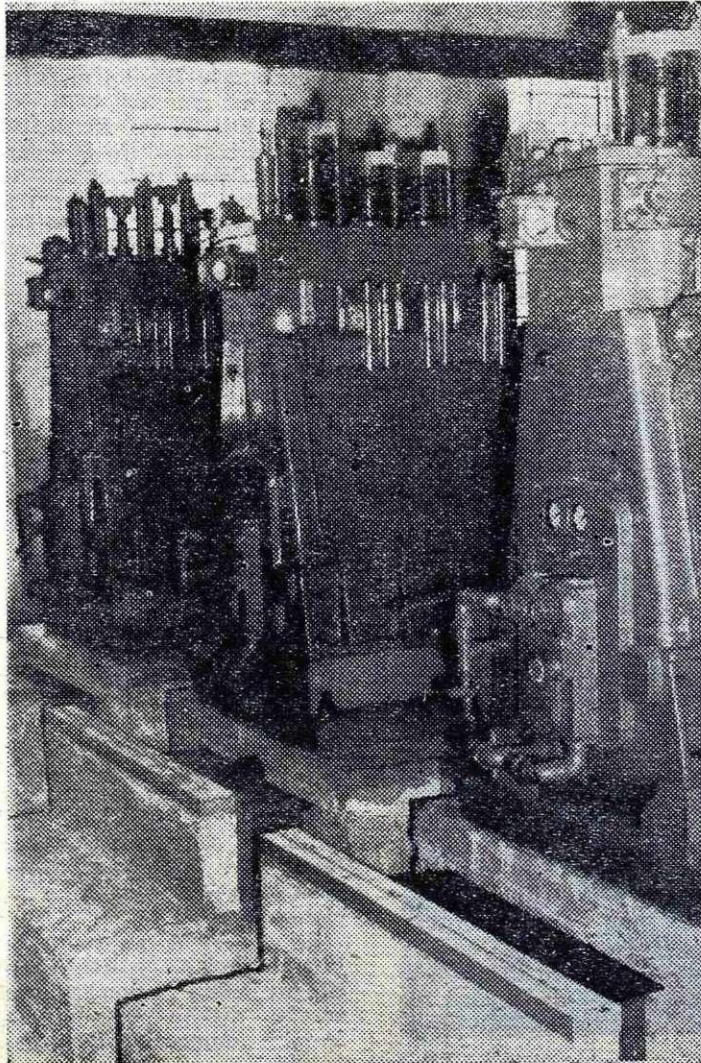
Naprava za odbrize kovarine v valjarni 2400 na Javorniku
