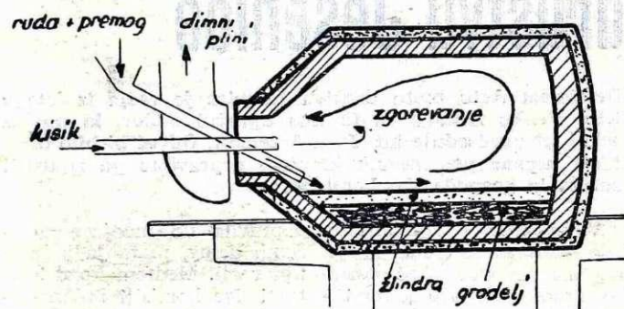
Skica konvertorja za proizvodnjo grodlja
