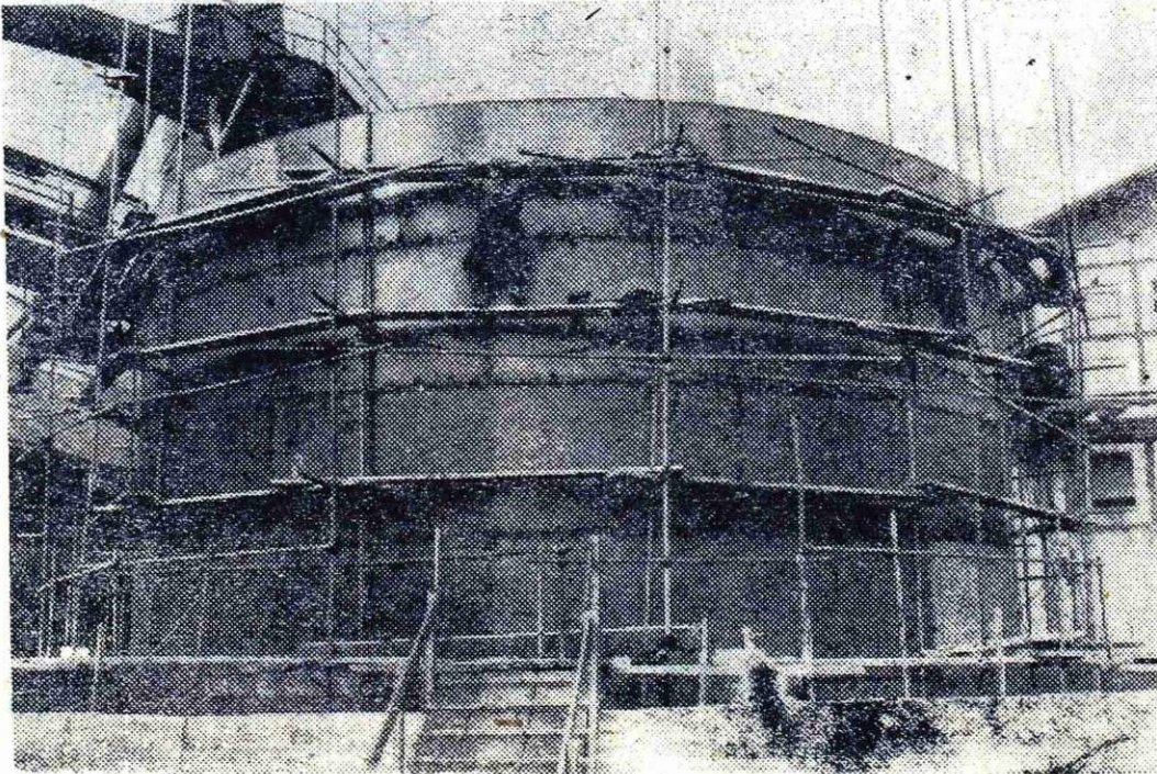
Gradnja mazutne postaje kljub slabim vremenskim prilikam lepo napreduje
