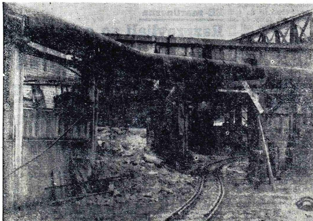
Tod bo vodila nova cesta k martinarni. Sedanji podvoz pod rakami že poglabljajo, da bodo lahko speljali novo cesto, po kateri bo martinarna dobivala opeko ne več v zaprtih normalnotirnih vagonih, temveč kar z vilicarji.
