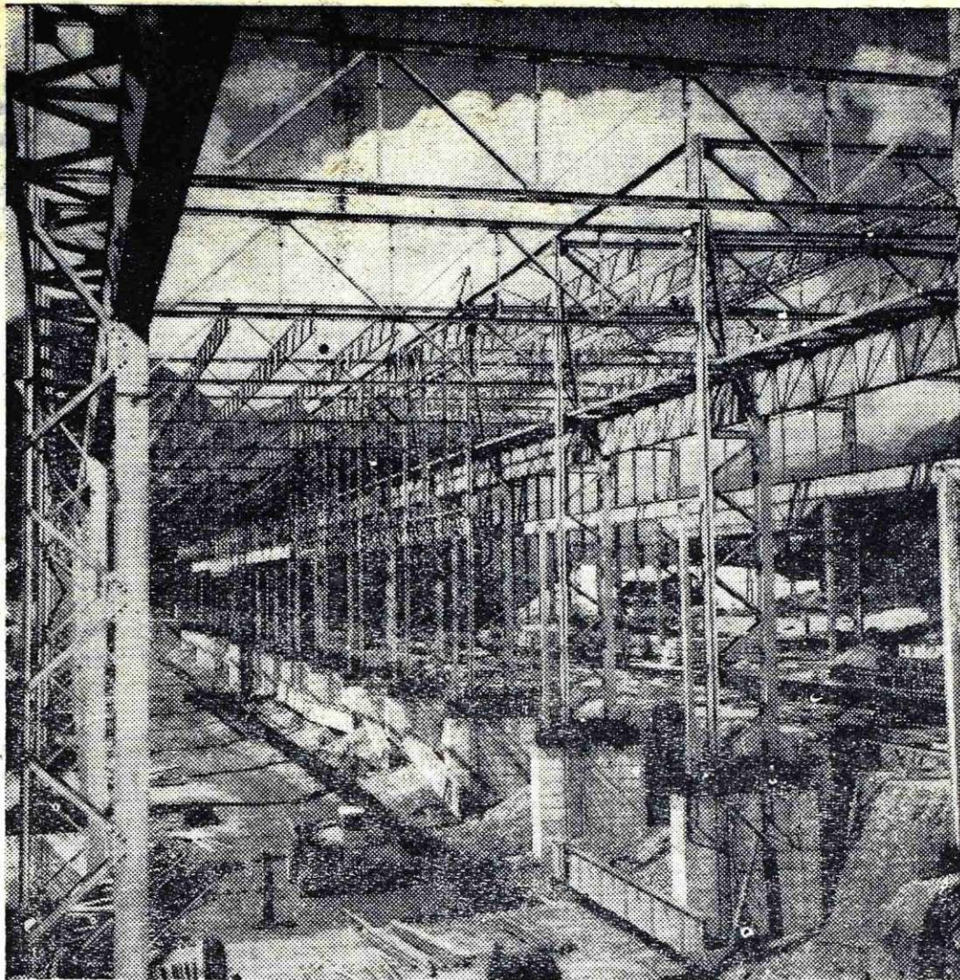
Na Belškem polju so začeli pokrivati strojnično halo in betonski temelje za strojne naprave
