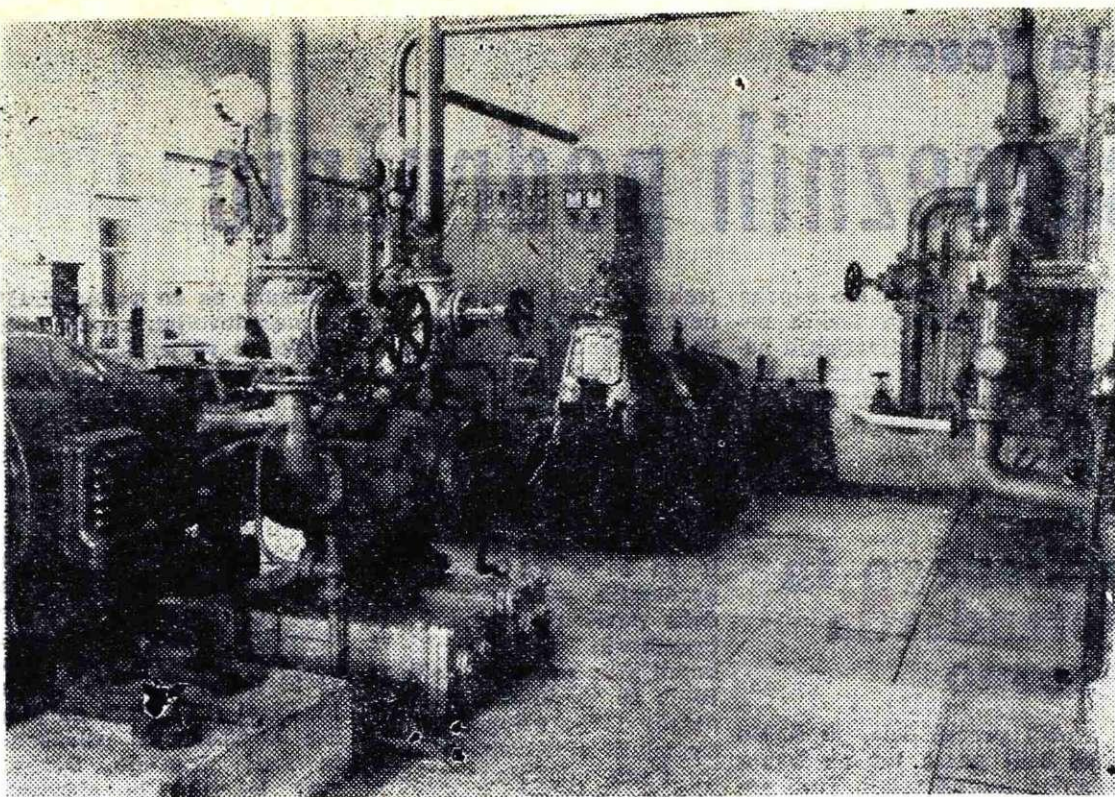
Na umetnem drsališču imajo dva kompresorja, ki so oba usposobili za obratovanje sami. Na sliki notranjost strojnice
