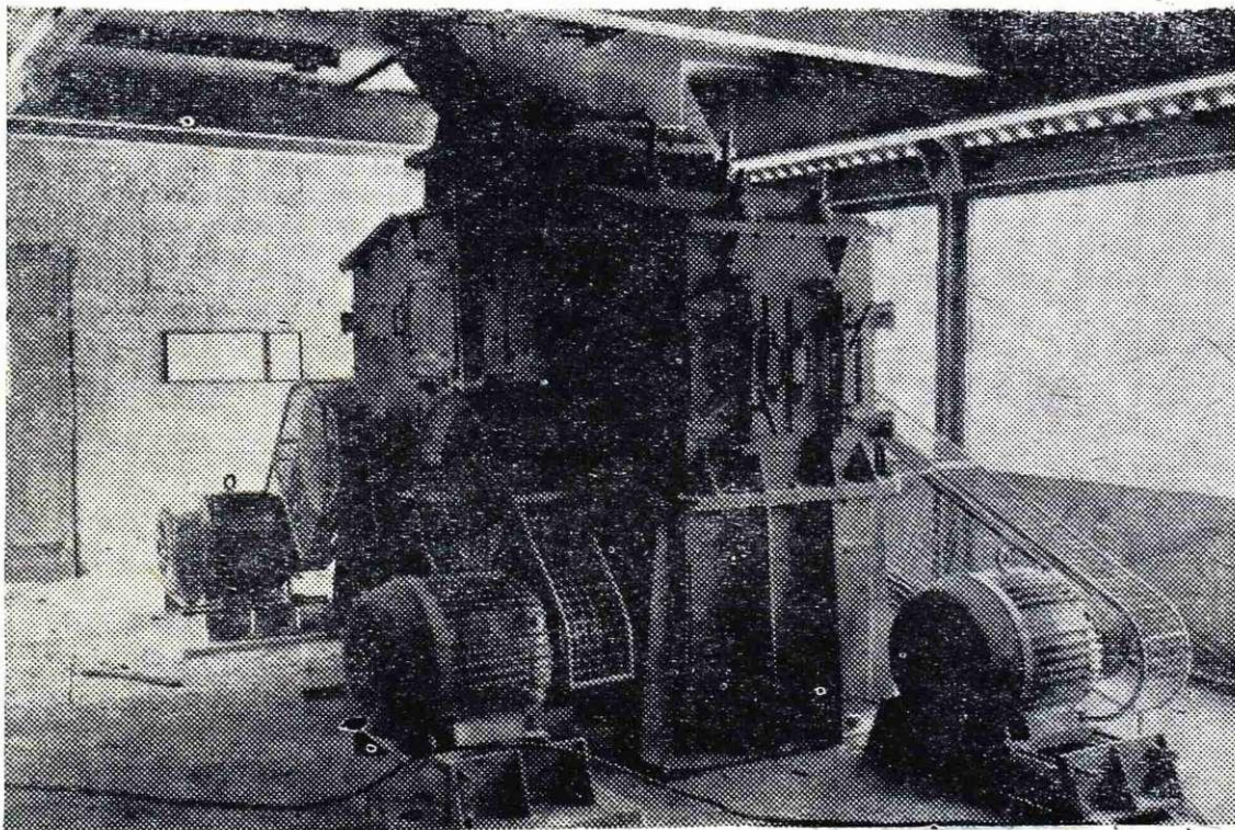
Udarni granulator za mletje apnenca na zrno pod 3 mm
