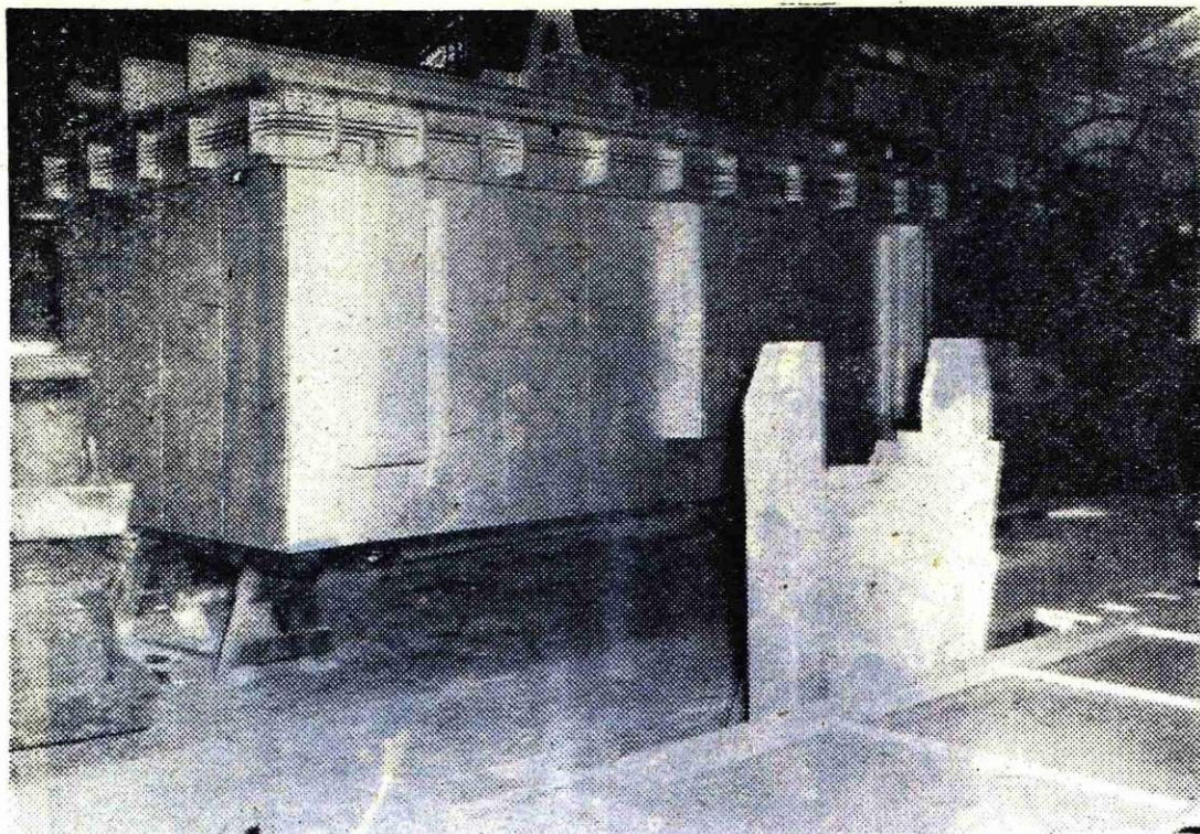
V adjustaži tanke pločevine na Iavorniku dela pri gradnji ASEA peči hitro napredujejo. Dela so v zaključni fazi in vgrajujejo merilne naprave.
