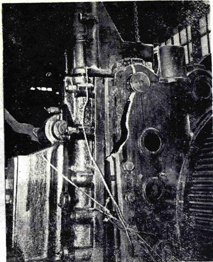
Na sliki je dobro vidna razpoka na ohišju, ki je nastala ob okvari na Sack škarnjah. Ker zaradi te okvare težka proga ni mogla obratovati, so opravili v določenem roku remont, četudi ni bil vnaprej planiran
