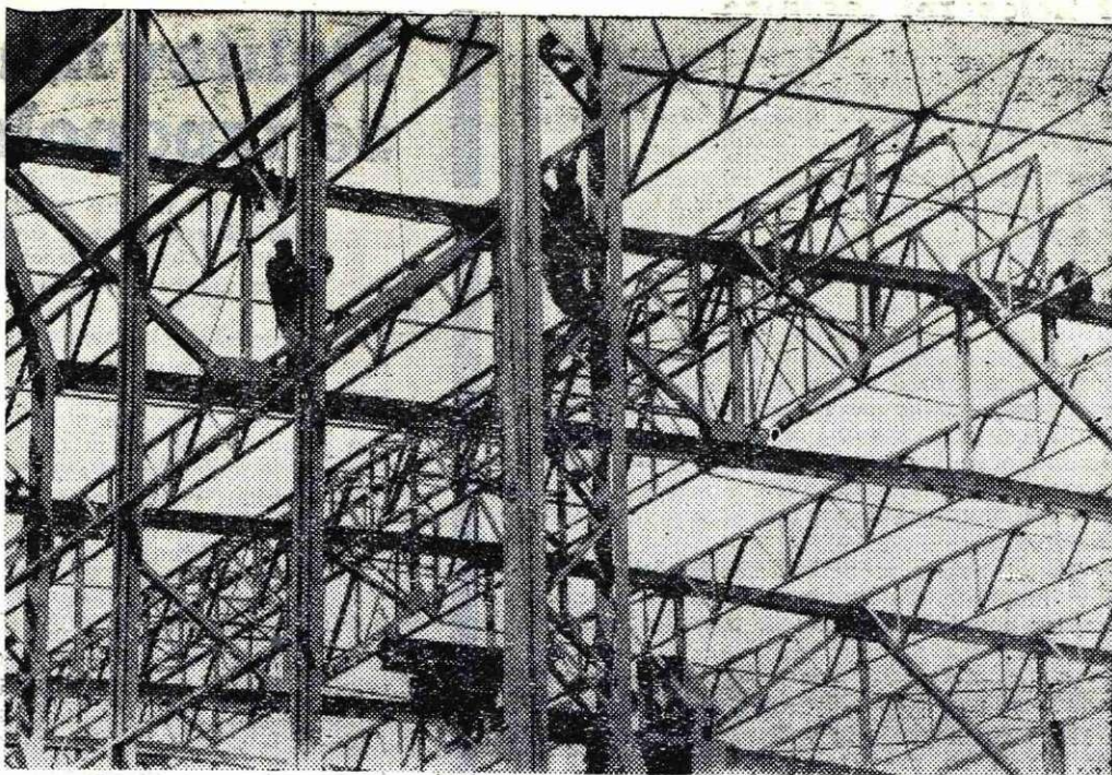
Dela pri montaži hal za valjarne na Belškem polju uspešno napredujejo in bodo zaključena pravočasno
