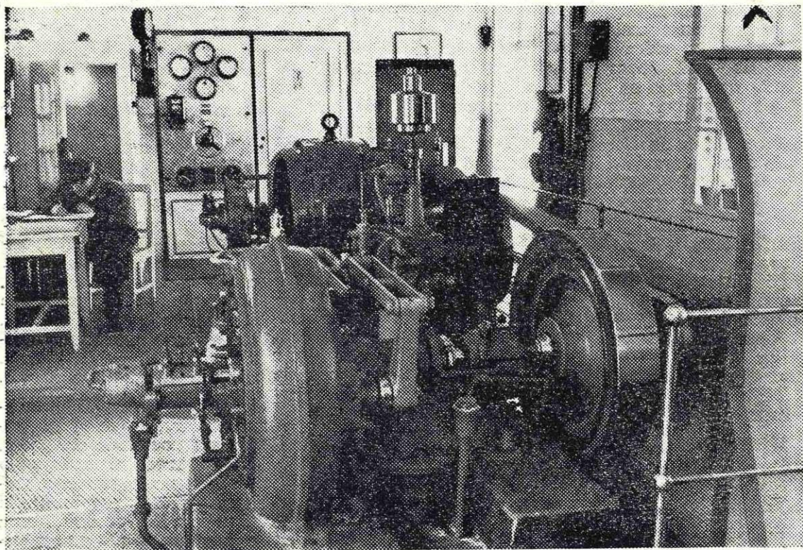
Tako izgleda notranjost strojnice poleg vodnega zbiralnika v Javorniškem rovtu.
