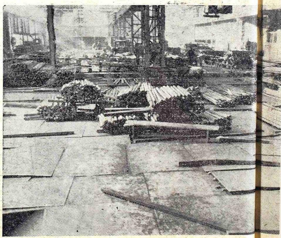
V adjustaži paličastega železa je zdaj dovolj prostora, ker lahko srednja obratujeta.
