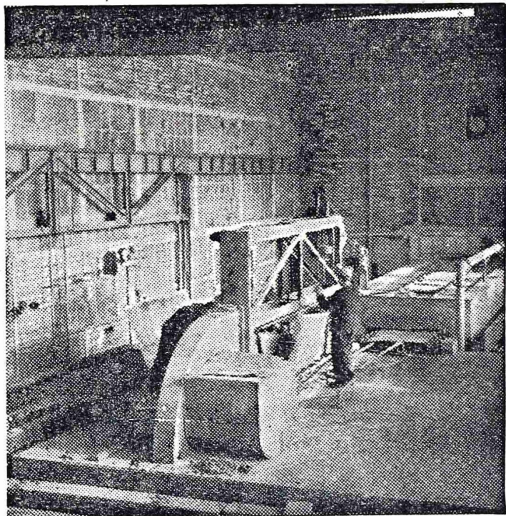
Sestavni del obrata Javornik II je pocinkovalnica za pocinkanje pločevine
