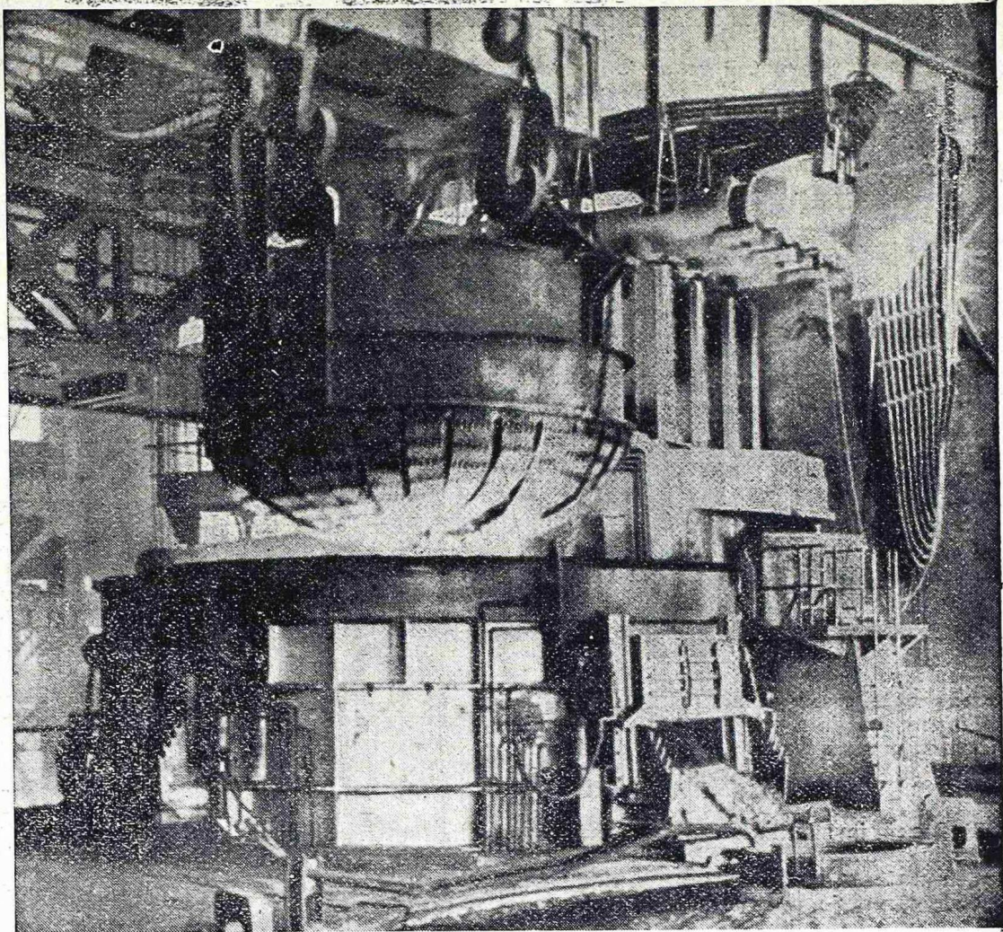
Moderne elektropeči zakladajo z vrha s košarami. Podobno peč, kot jo vidite na sliki, bomo dobili po sedanjih načrtih tudi v našo železarno
