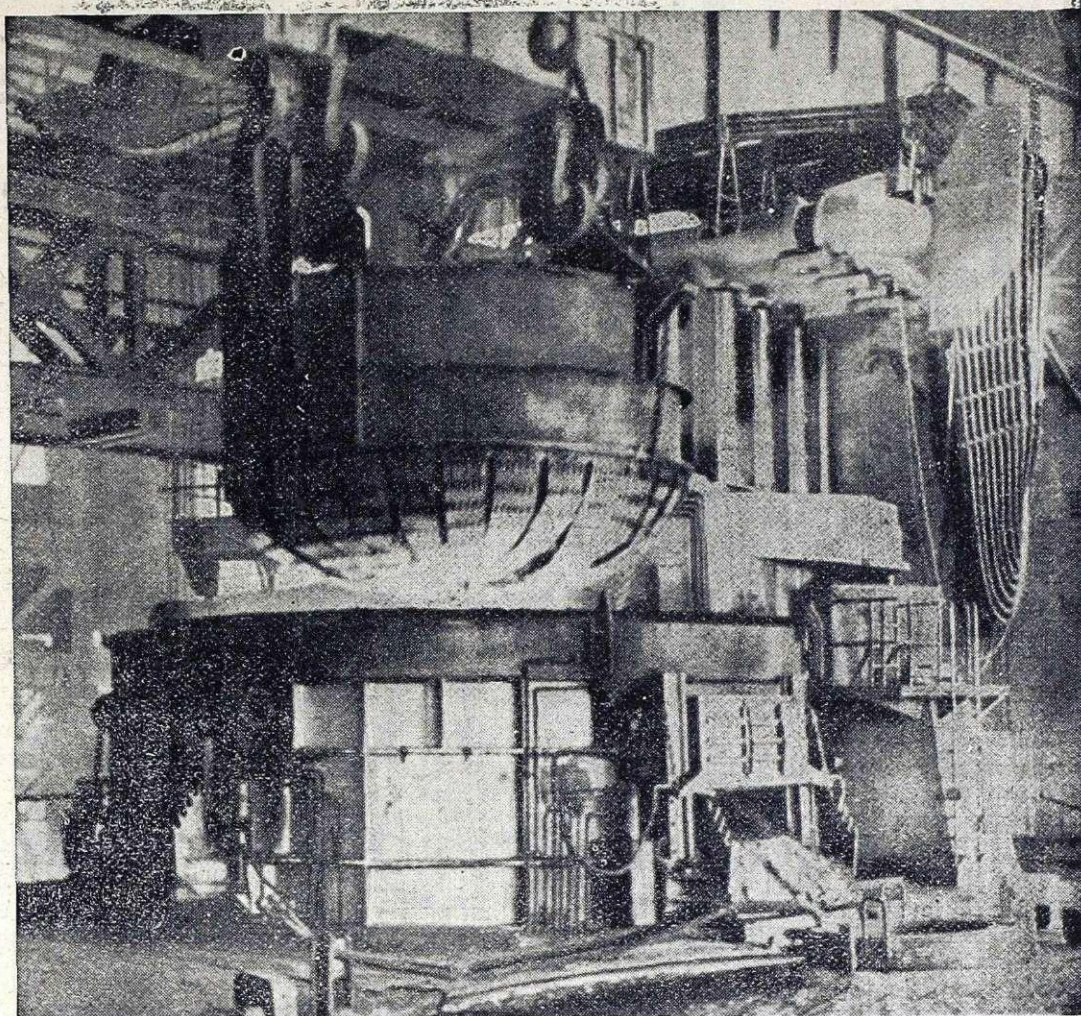
Modernne elektropeči zakladajo z vrha s košarami. Podobno peč, kot jo vidite na sliki, bomo dobili po sedanjih načrtih tudi v našo železarno
