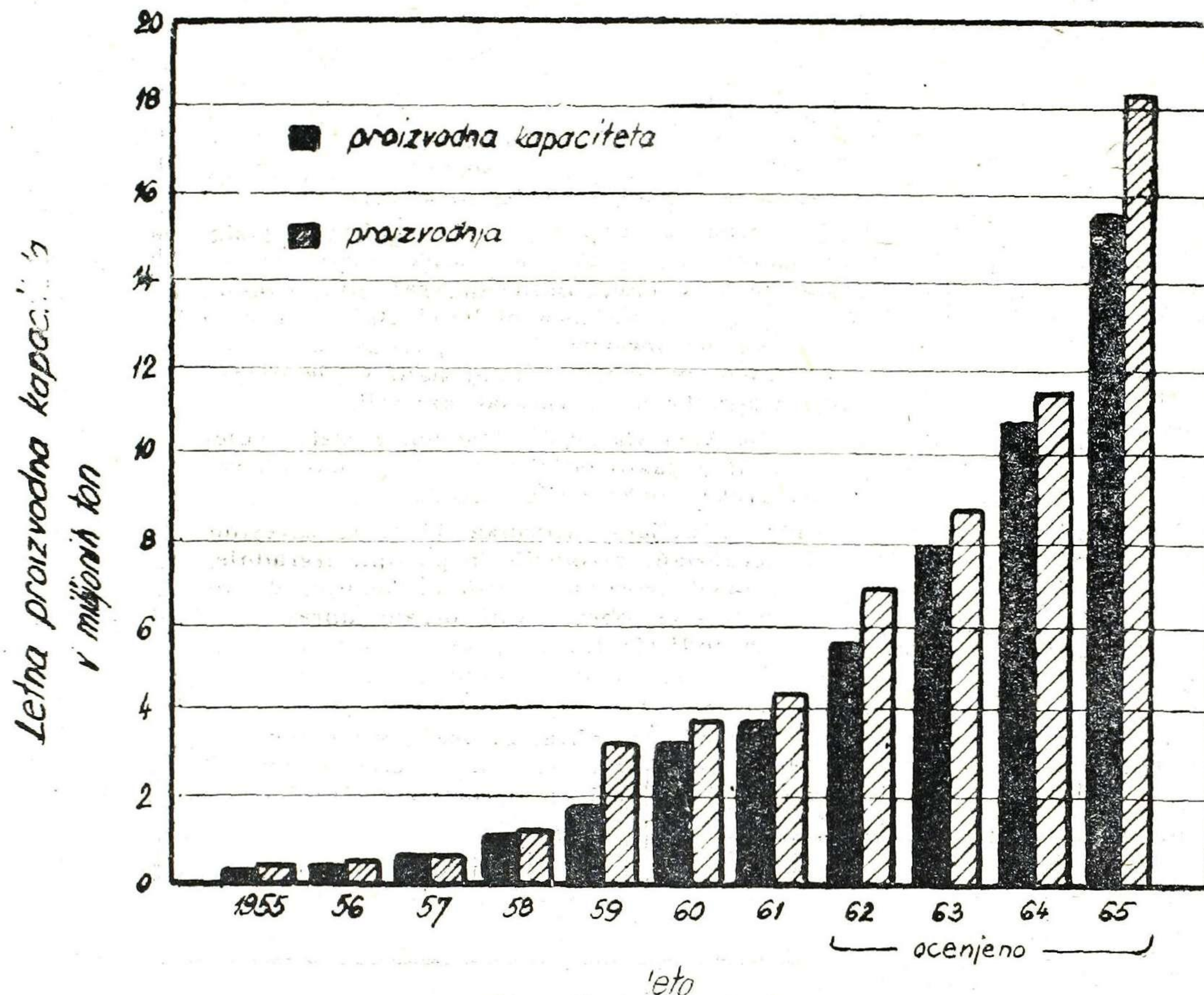
Kapaciteta in proizvodnja kisikovih konvertorjev v ZDA
