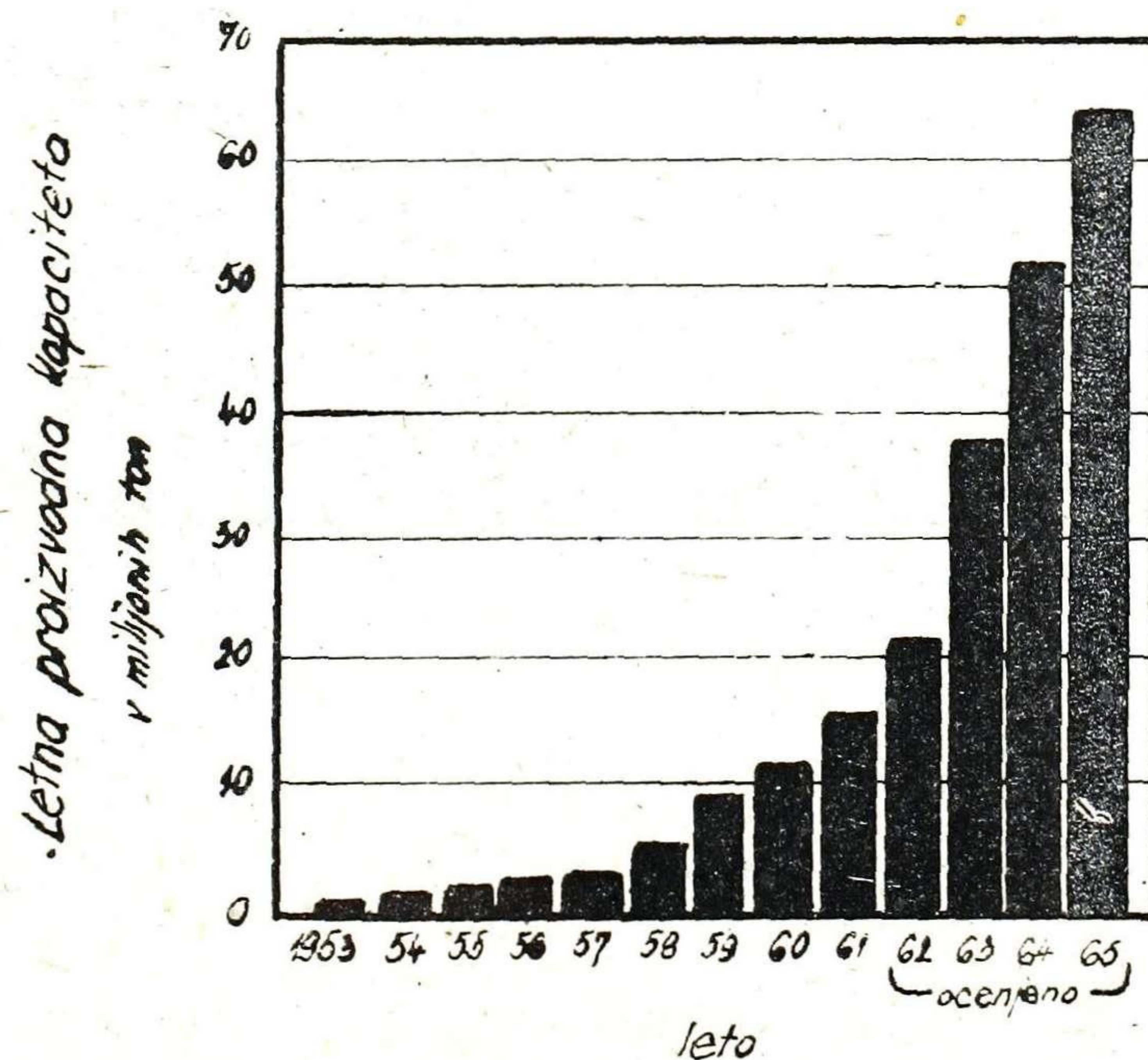
Svetovna proizvodnja jekla v kisikovih konvertorjih
