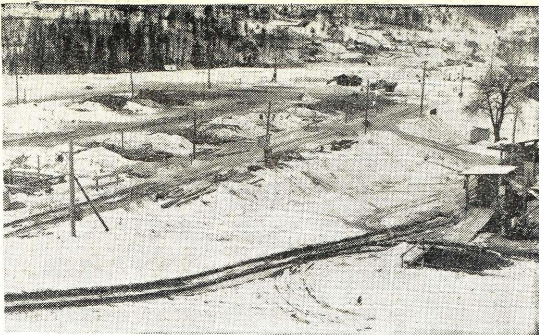
Pred kratkim so začeli z izkopom temeljev za stripper halo v sklopu novih valjarn na Belškem polju
