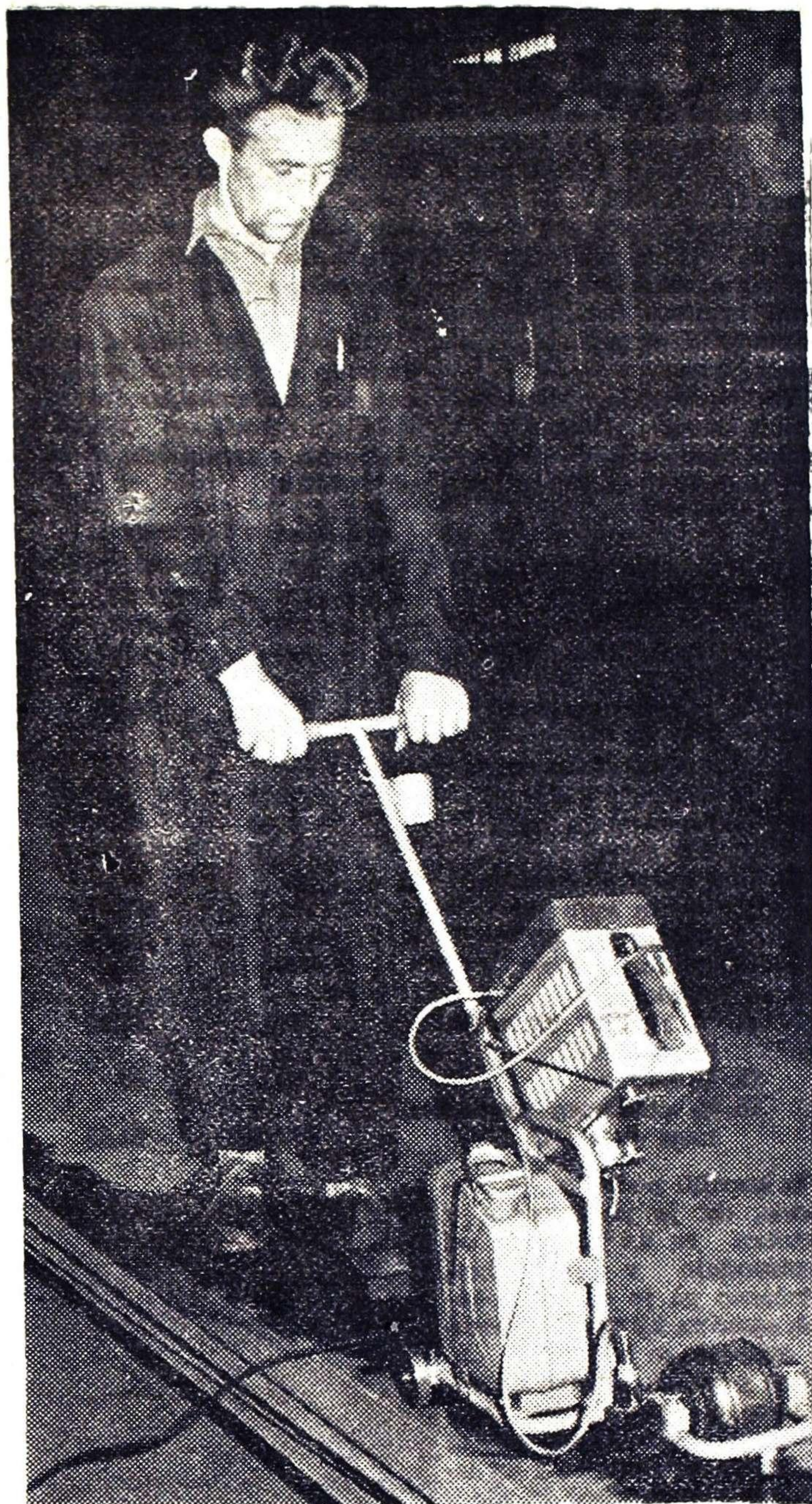
Kontinuirano preiskovanje pločevine z ultra zvokom
