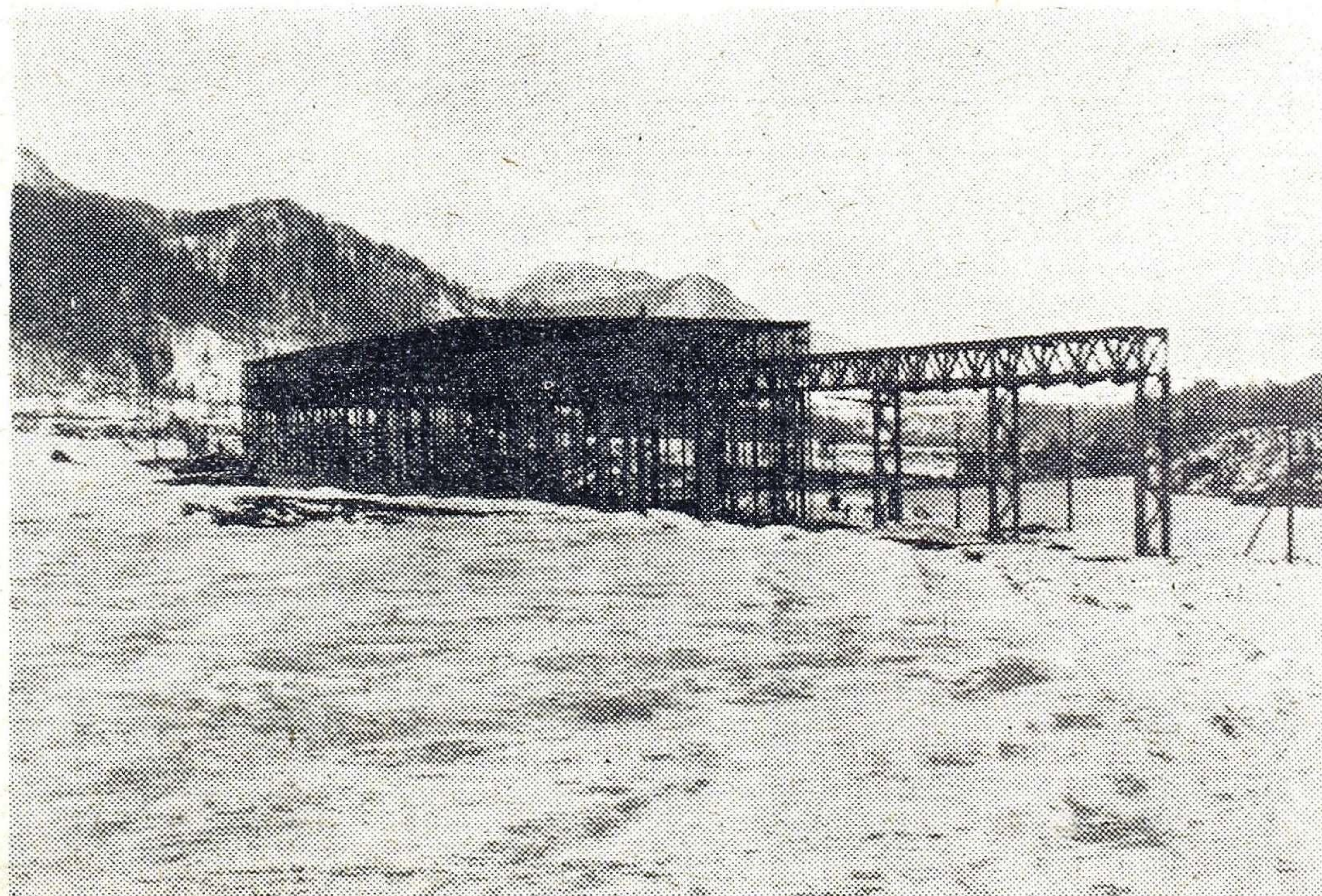
Na Belškem polju hitijo z deli pri gradnji hale za vzdrževanje, da bo pravočasno pripravljena za vskladiščenje novih naprav in opreme, ko bo prispela
