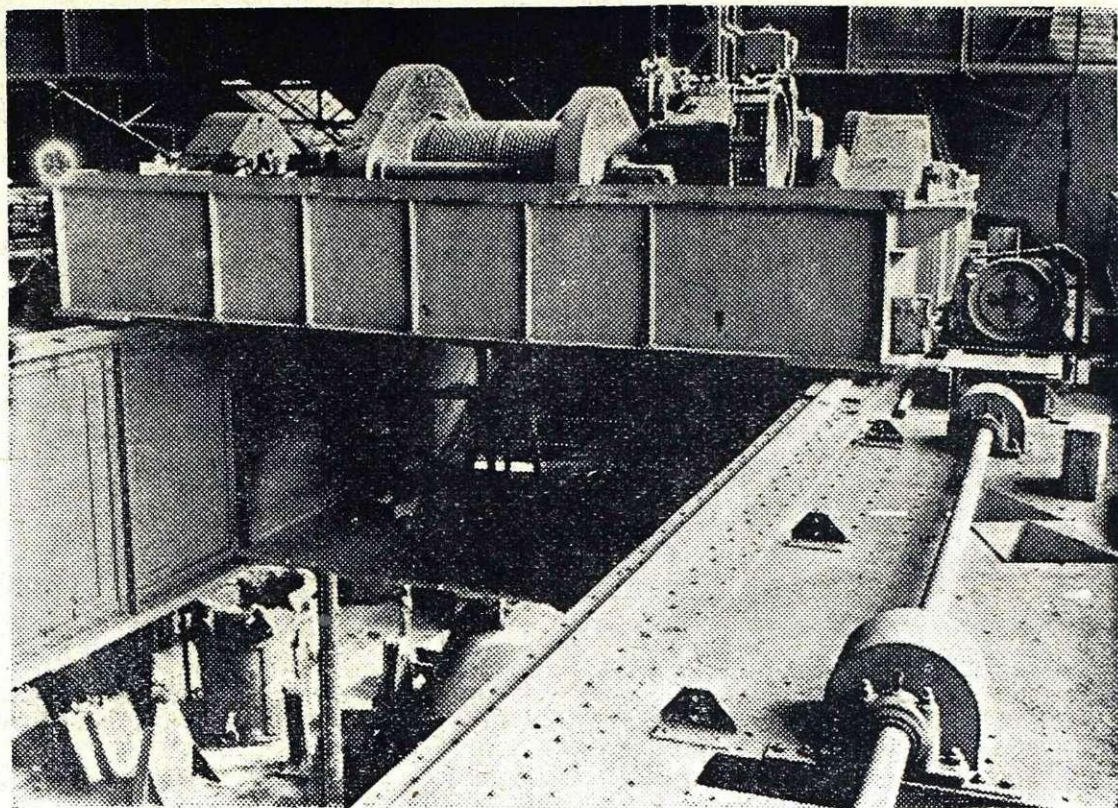
Detalj z novega livnega žerjava v martinarni. — Predvidena sredstva bodo prekoračena verjetno za 24,3 milijona dinarjev
