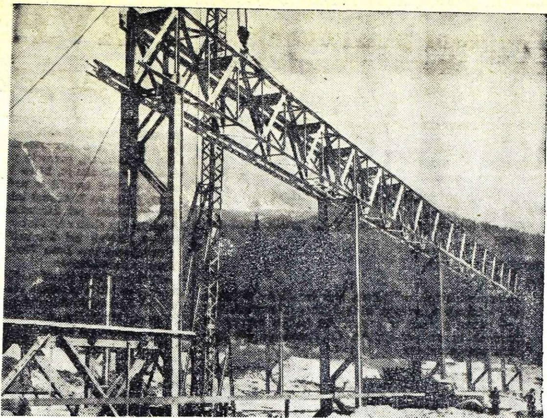
Montažna dela pri hali za vzdrževanje na Belškem polju lepo napredujejo. Navpične stebre že povezujejo vzdolžni nosilci. Toda z deli bo treba pohiteti, da bo hala pravočasno pripravljena za sprejem novih naprav, ki bodo do montaže vskladiščene v tej hali
