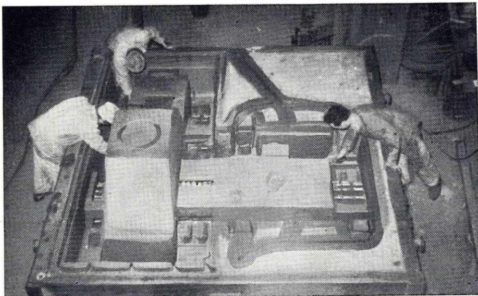
Pogled z žerjava na kalup ohišja za »SIEMAG« foto Torkar
