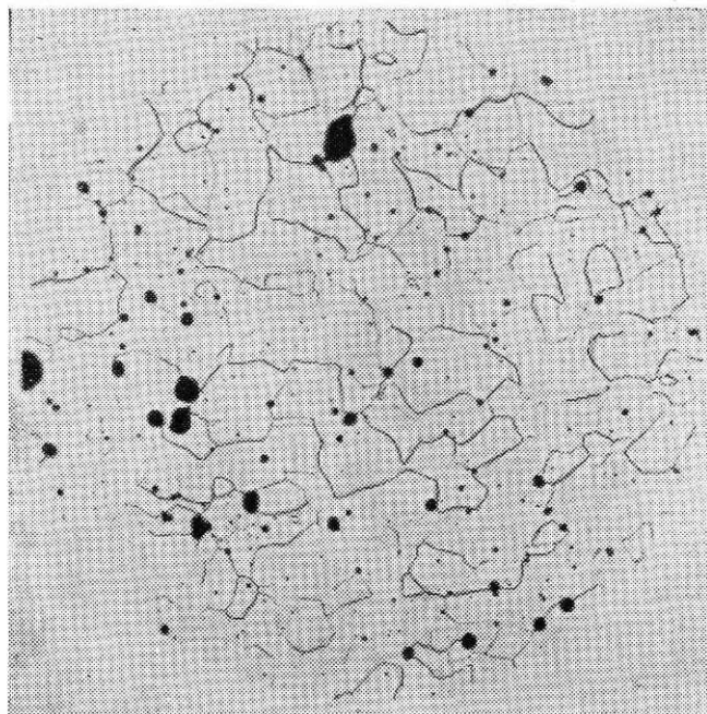
Metalografski izgled železne konice (povečava 100 X)
