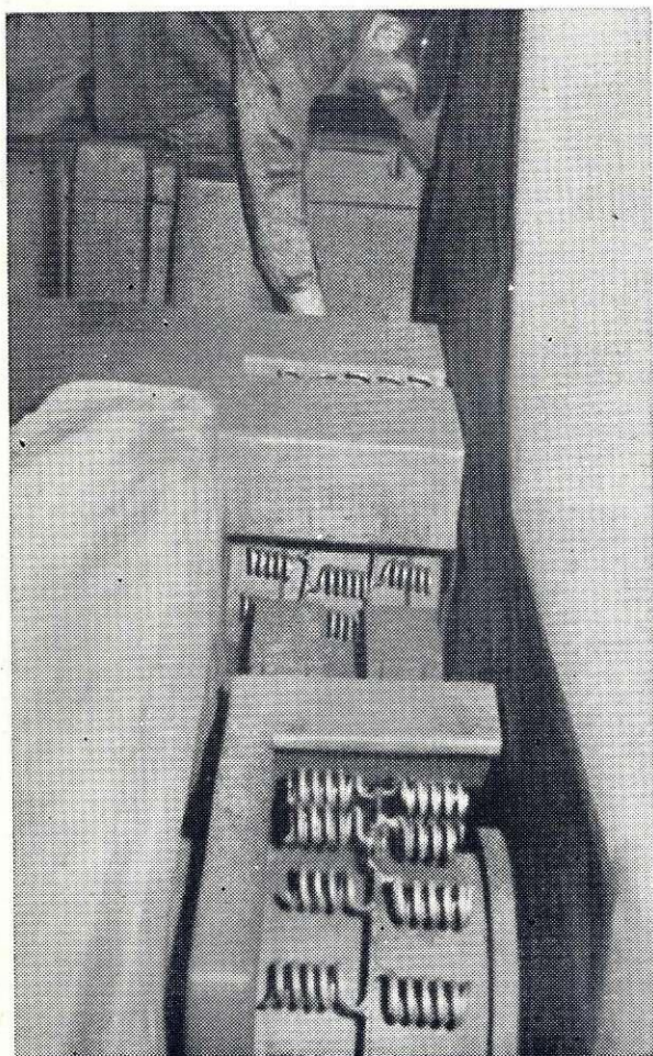
Del jeder in hladilnih vložkov v kalupu ohišja za »SIEMAG« foto Torkar
